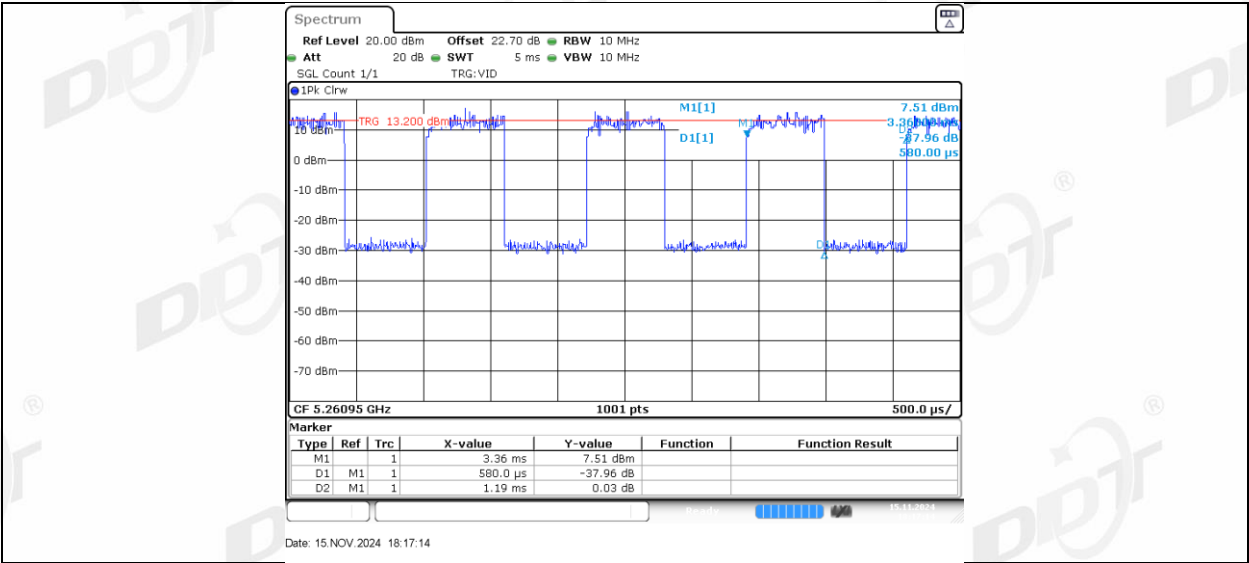
11AX20MIMO_Ant2_5260_26Tone_RU8
