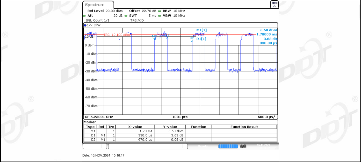
11AX20MIMO_Ant2_5260_52Tone_RU39
