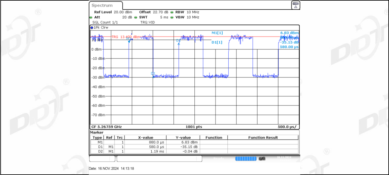
11AX20MIMO_Ant2_5260_52Tone_RU37
