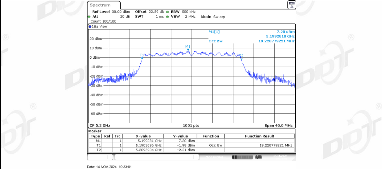
11AX20MIMO_Ant2_5200
