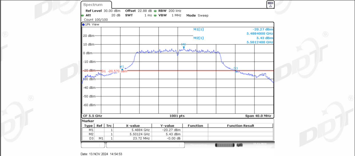
11AC20MIMO_Ant2_5500
