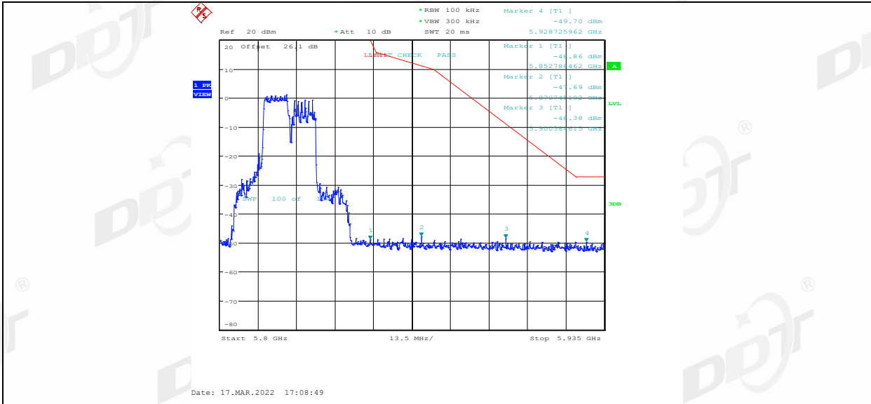
11AX20MIMO_Ant2_5825_106Tone_RU54
