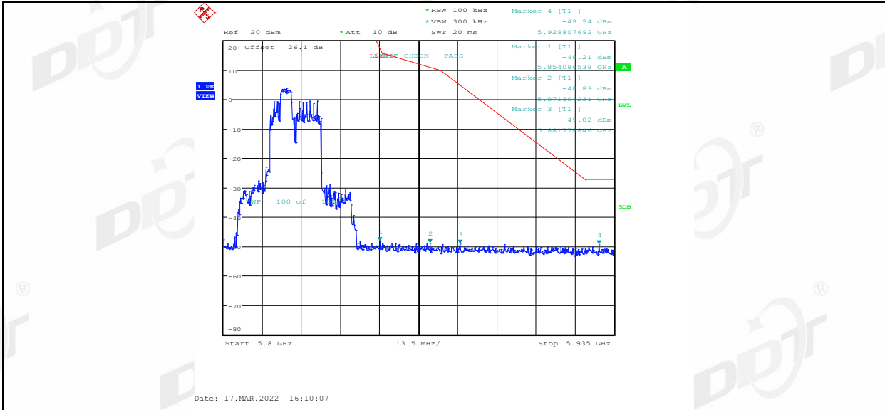
11AX20MIMO_Ant2_5825_52Tone_RU39
