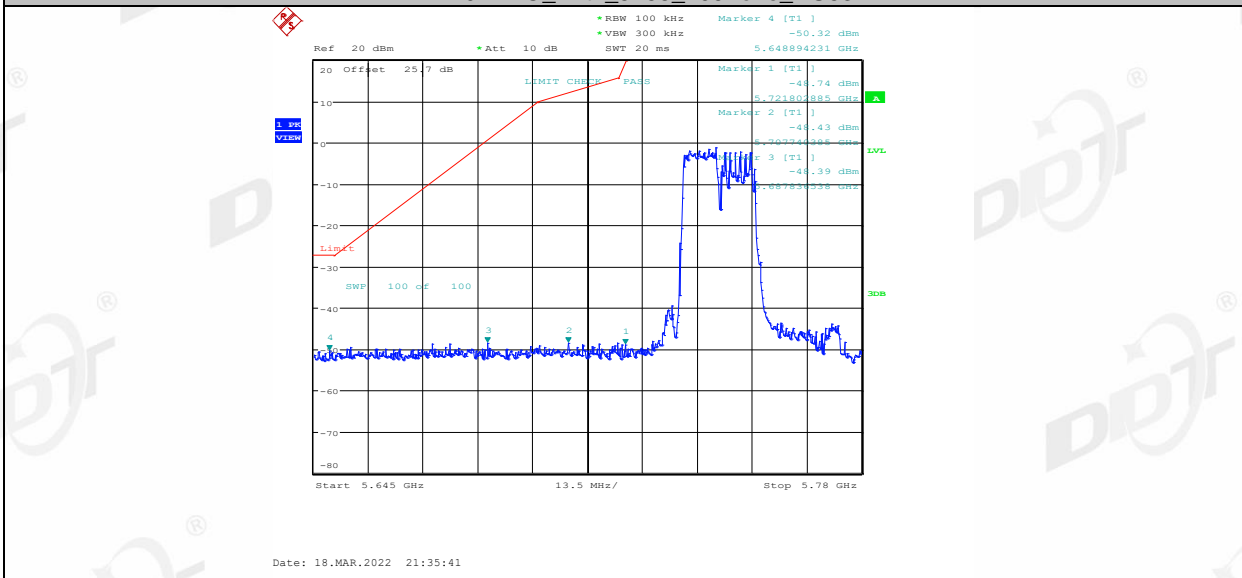
11AX40MIMO_Ant1_5755_106Tone_RU54
