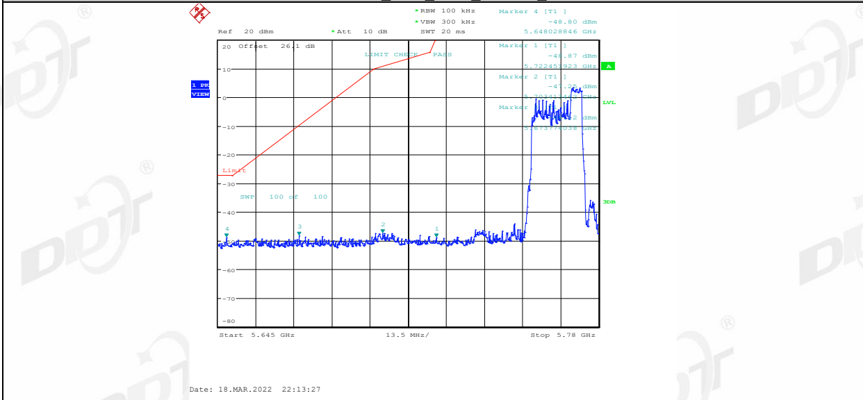
11AX40MIMO_Ant2_5755_106Tone_RU53
