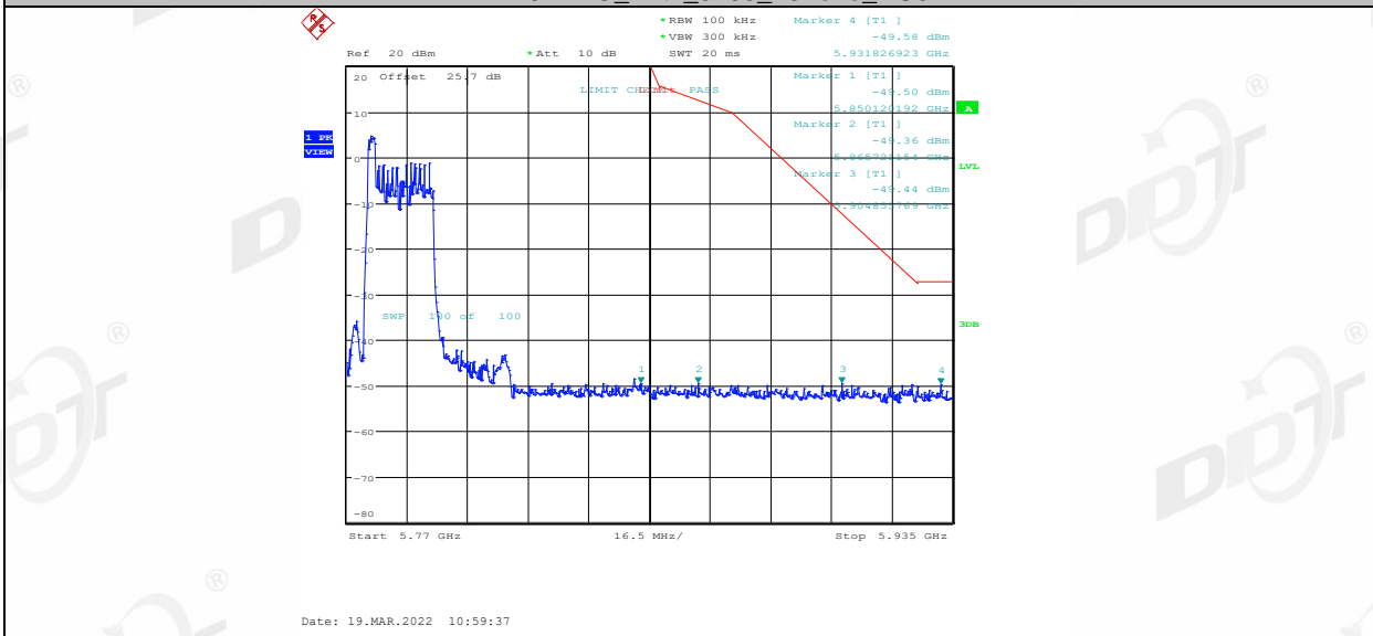
11AX40MIMO_Ant1_5795_26Tone_RU8
