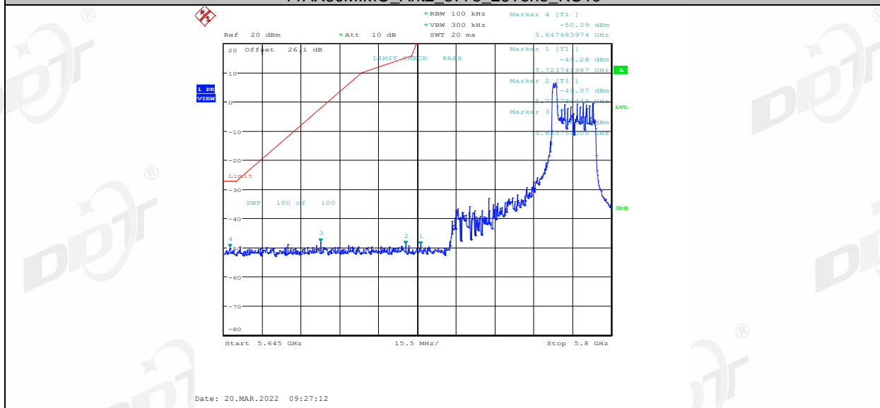
11AX80MIMO_Ant2_5775_26Tone_RU19
