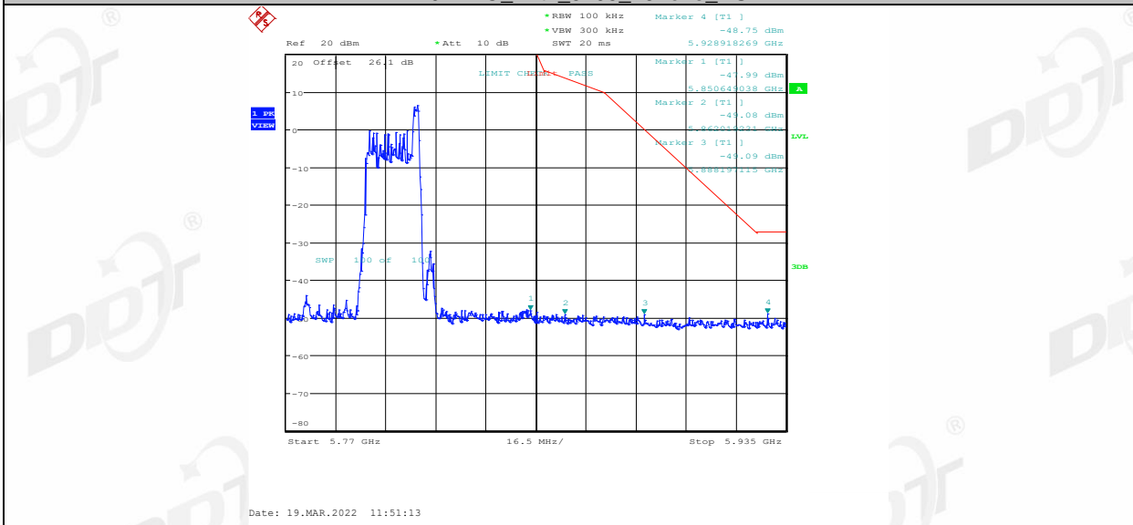
11AX40MIMO_Ant2_5795_52Tone_RU37
