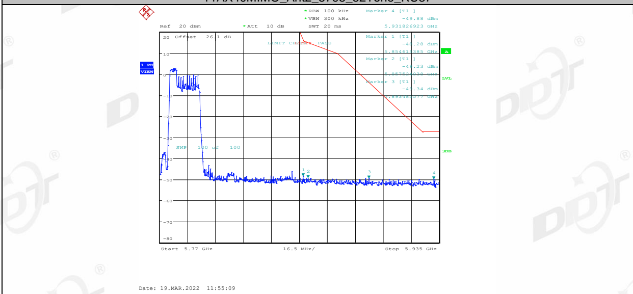
11AX40MIMO_Ant2_5795_52Tone_RU40
