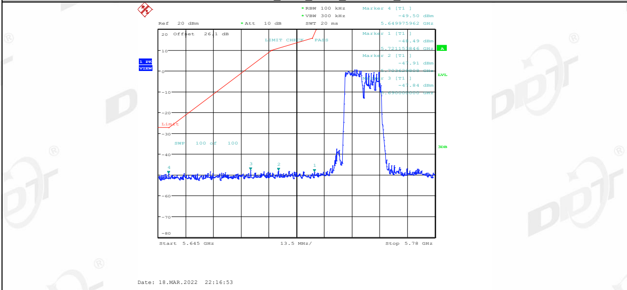
11AX40MIMO_Ant2_5755_106Tone_RU54
