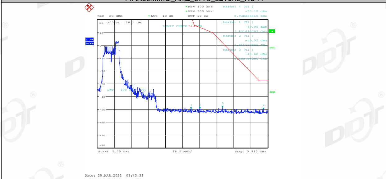
11AX80MIMO_Ant2_5775_52Tone_RU52
