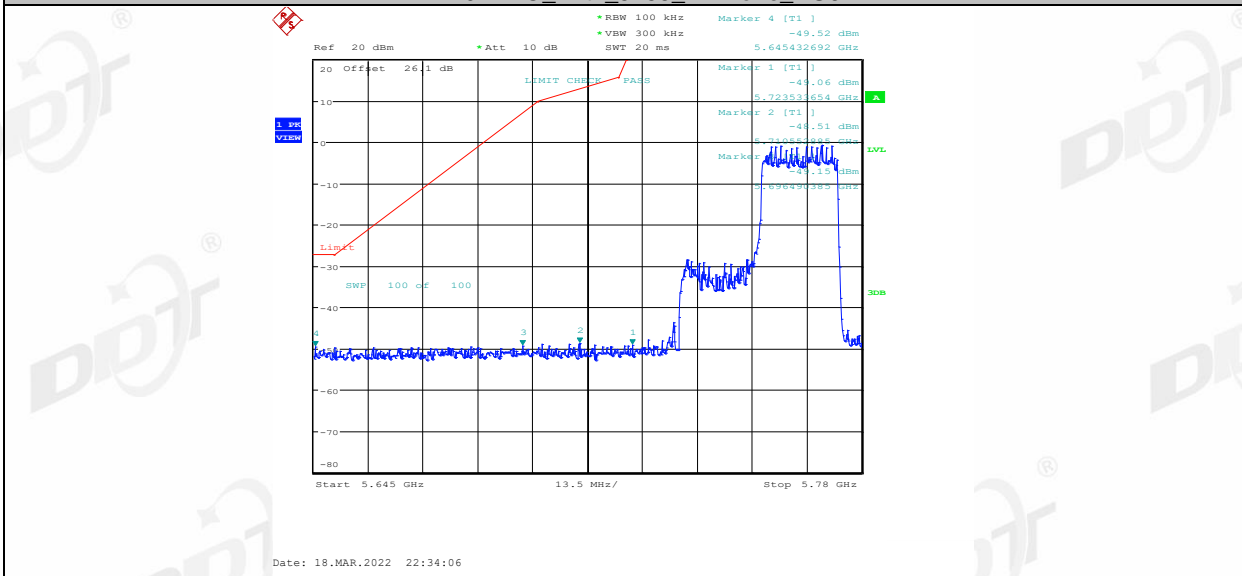
11AX40MIMO_Ant1_5795_26Tone_RU0
