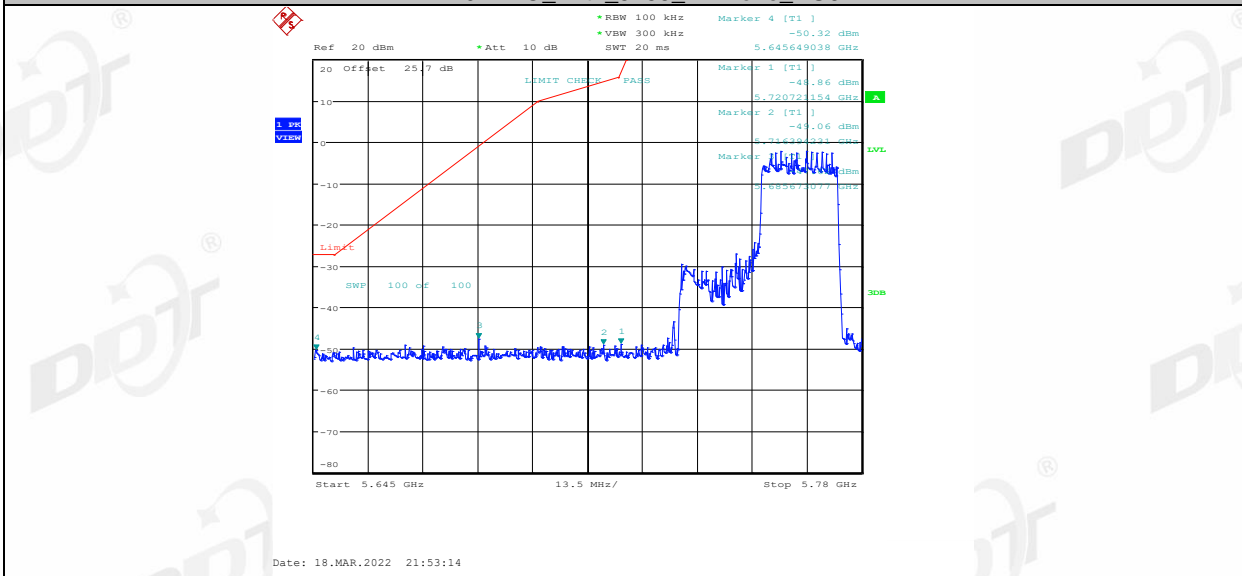
11AX40MIMO_Ant2_5755_26Tone_RU0
