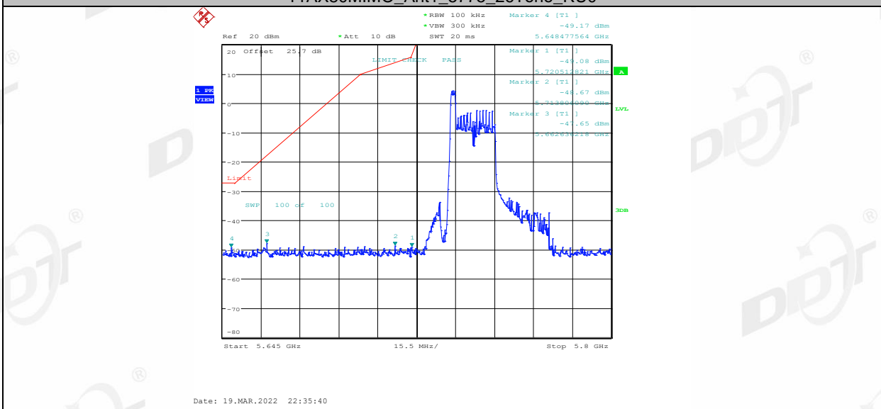
11AX80MIMO_Ant1_5775_26Tone_RU0
