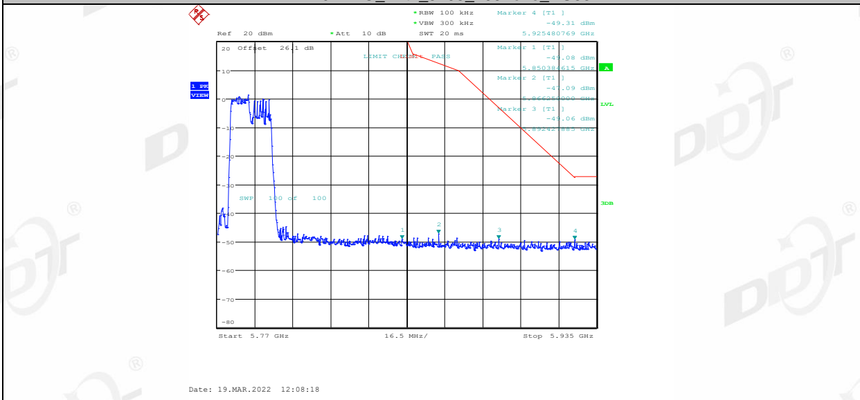
11AX40MIMO_Ant2_5795_106Tone_RU54
