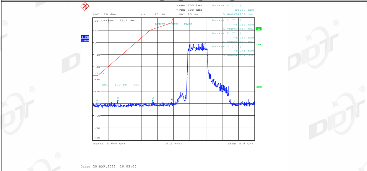
11AX80MIMO_Ant2_5775_242Tone_RU61
