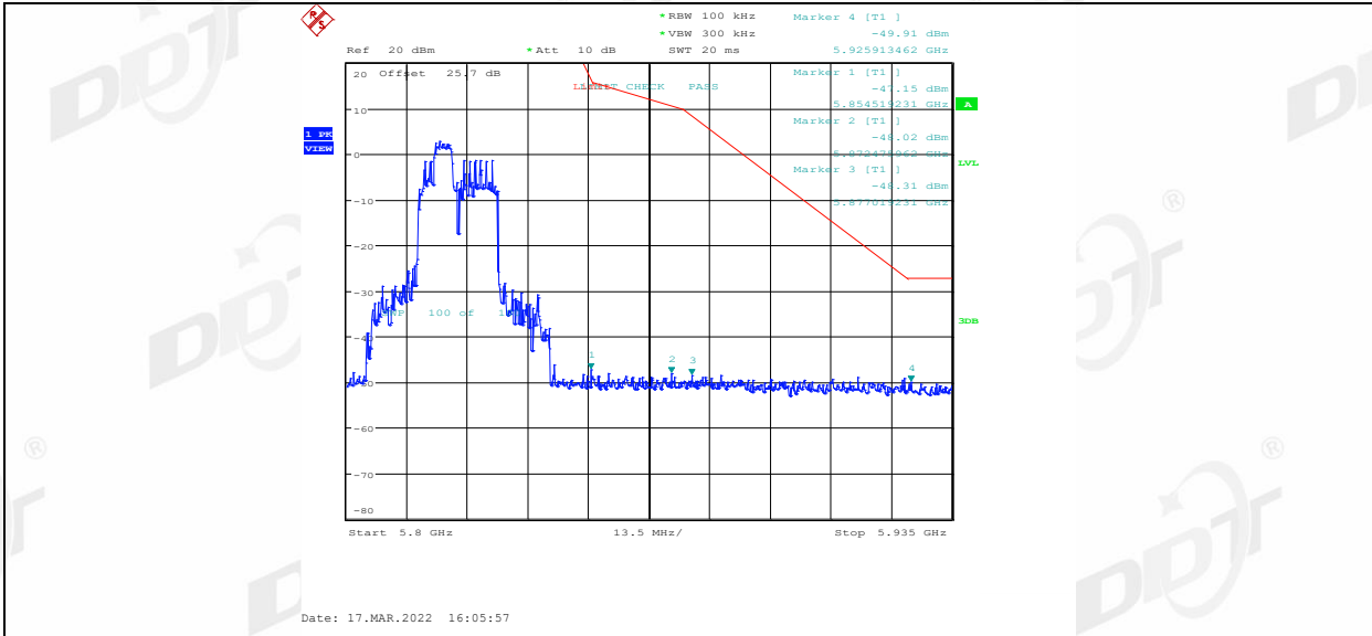
11AX20MIMO_Ant1_5825_52Tone_RU39
