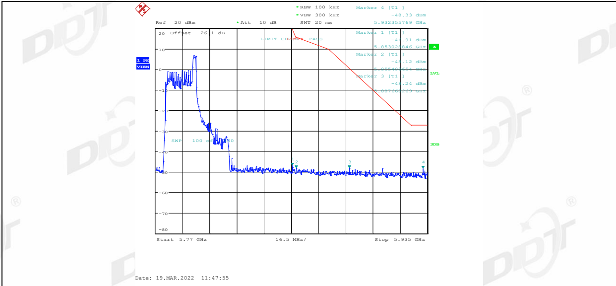
11AX40MIMO_Ant2_5795_26Tone_RU17
