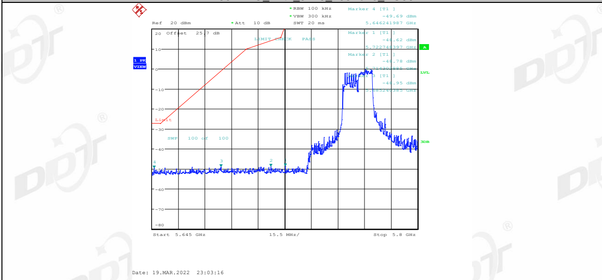
11AX80MIMO_Ant1_5775_106Tone_RU56
