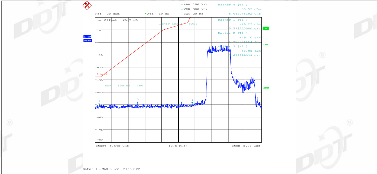
11AX40MIMO_Ant1_5755_242Tone_RU62
