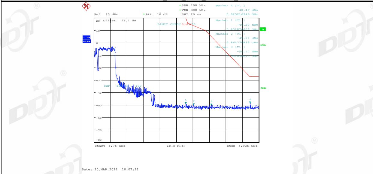
11AX80MIMO_Ant2_5775_242Tone_RU62
