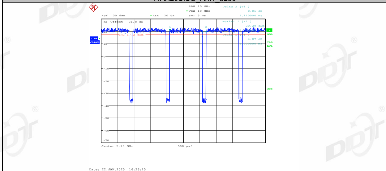
11AX20SISO_Ant1_5320
