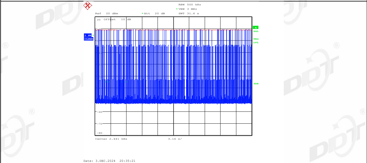
3DH1_Ant1_Hop
