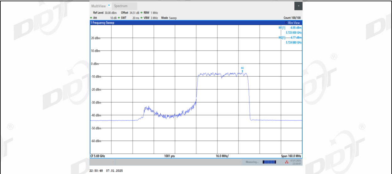
11AX80MIMO_Ant2_5690_UNII-2C_484Tone_RU65
