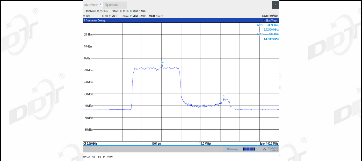
11AX80MIMO_Ant2_5690_UNII-2C_484Tone_RU66
