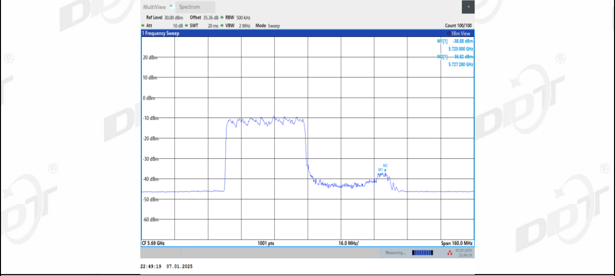
11AX80MIMO_Ant2_5690_UNII-3_484Tone_RU66
