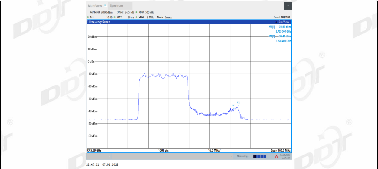
11AX80MIMO_Ant1_5690_UNII-3_484Tone_RU66
