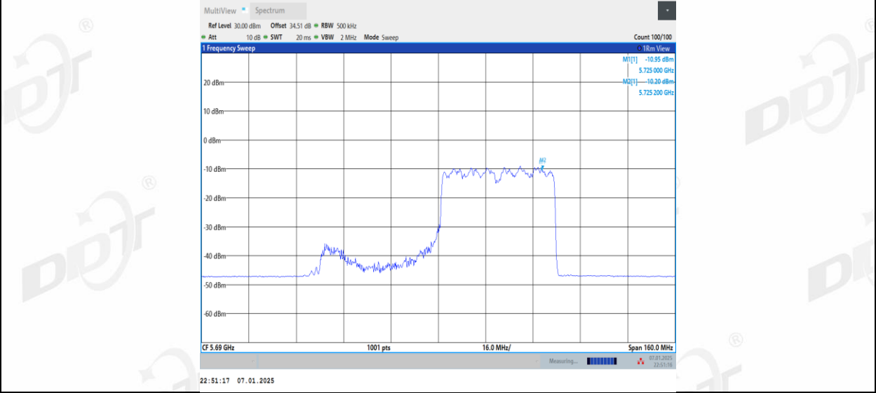
11AX80MIMO_Ant2_5690_UNII-3_484Tone_RU65
