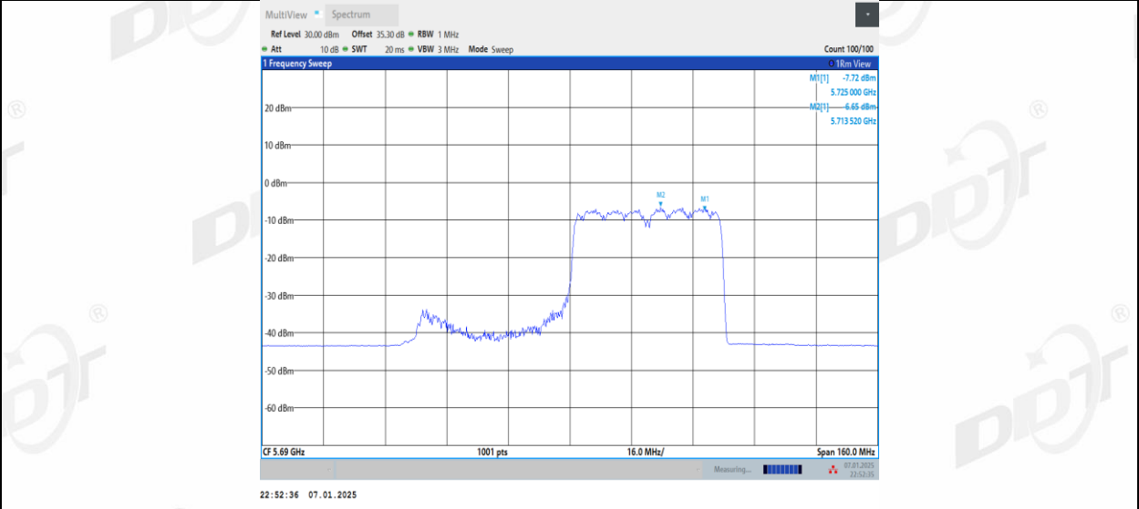
11AX80MIMO_Ant1_5690_UNII-3_484Tone_RU65
