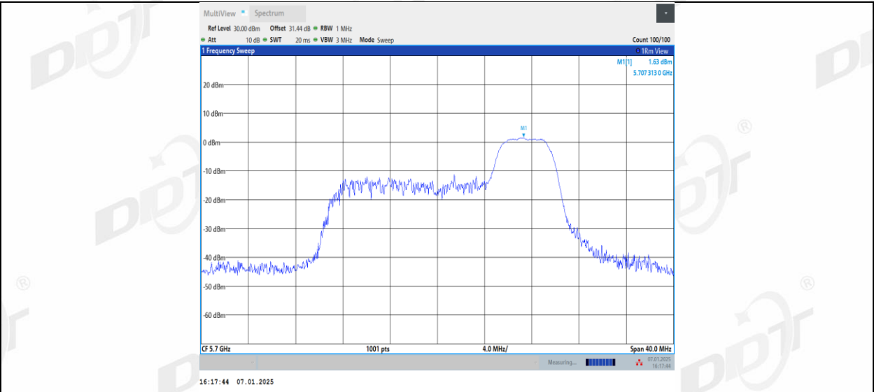
11AX20MIMO_Ant2_5700_106Tone_RU53
