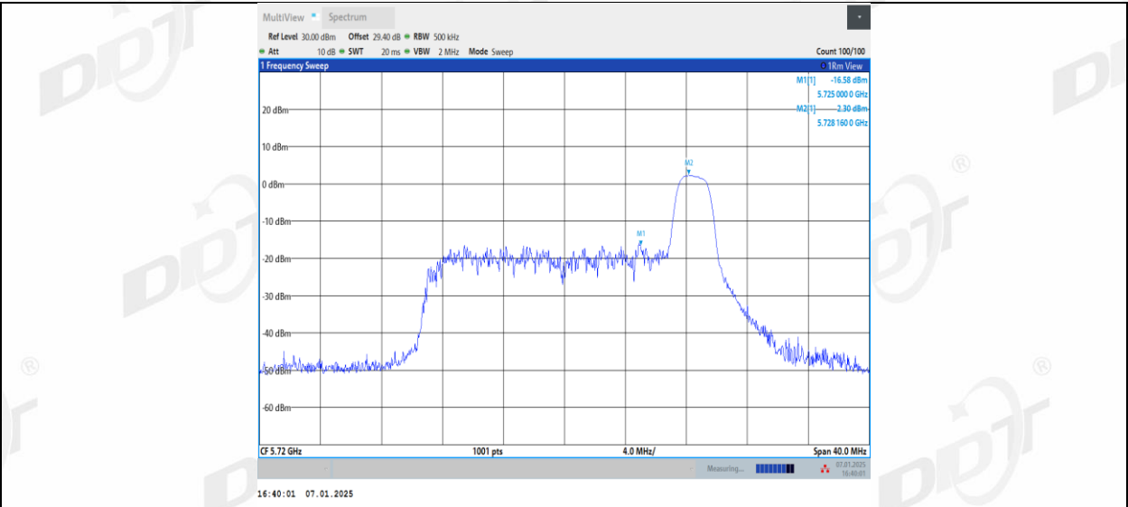
11AX20MIMO_Ant1_5720_UNII-3_52Tone_RU37
