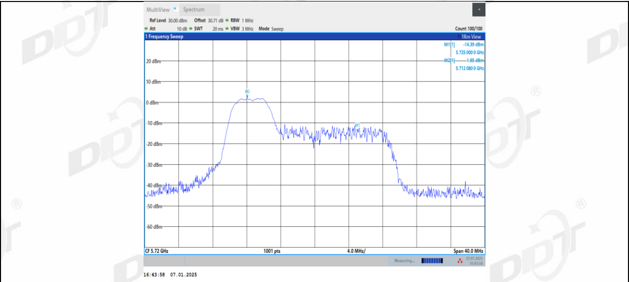
11AX20MIMO_Ant1_5720_UNII-2C_52Tone_RU39
