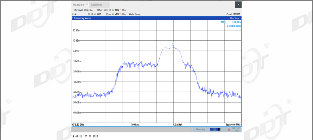
11AX20MIMO_Ant1_5320_52Tone_RU40
