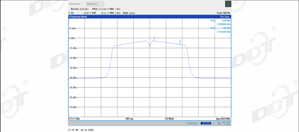
11N40MIMO_Ant1_5710_UNII-3
