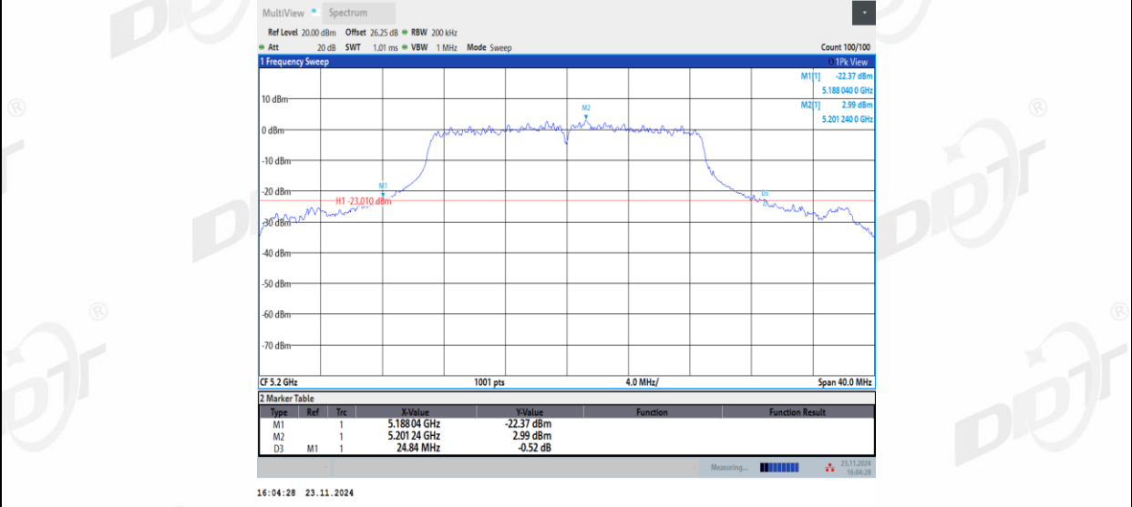
11AC20MIMO_Ant2_5200
