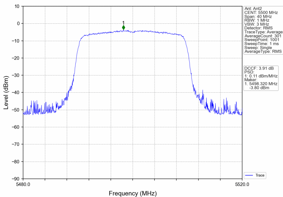
802.11ax(HEW20)_LCH_5500MHz_RU242_Left_Ant2_NTNV
