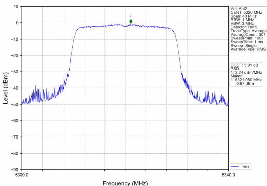
802.11ax(HEW20)_HCH_5320MHz_RU242_Left_Ant2_NTNV
