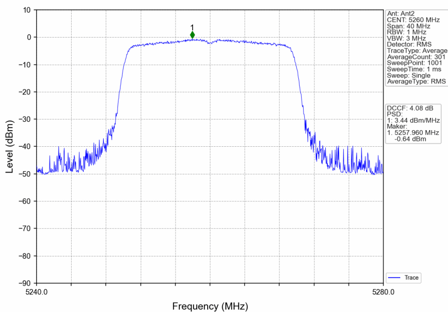
802.11ax(HEW20)_LCH_5260MHz_RU242_Left_Ant2_NTNV
