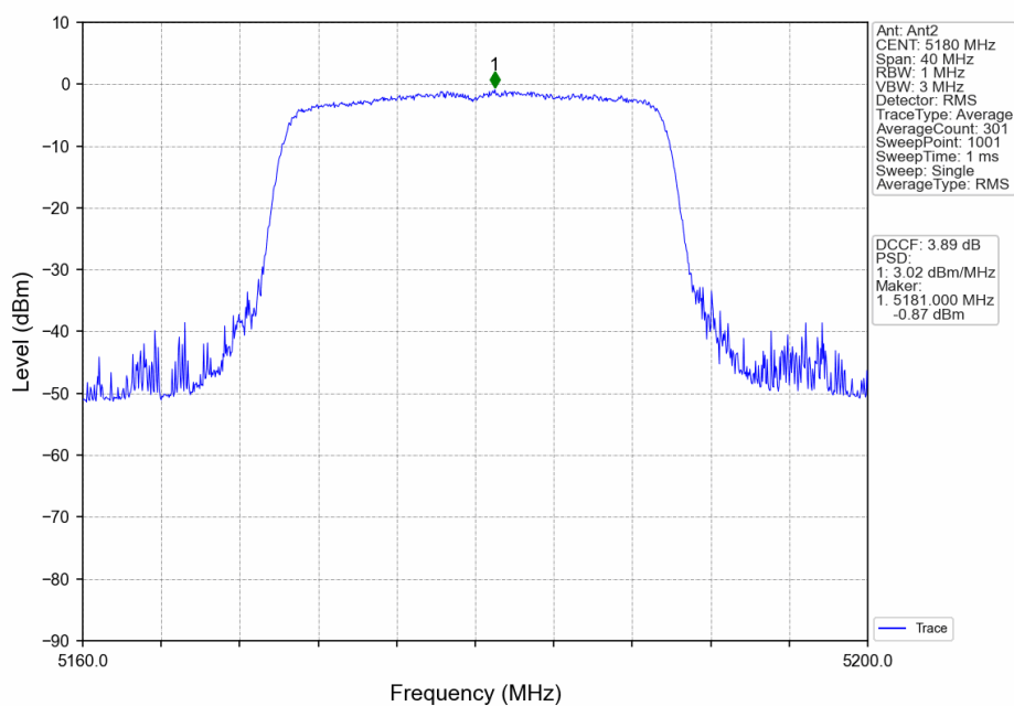
802.11ax(HEW20)_LCH_5180MHz_RU242_Left_Ant2_NTNV
