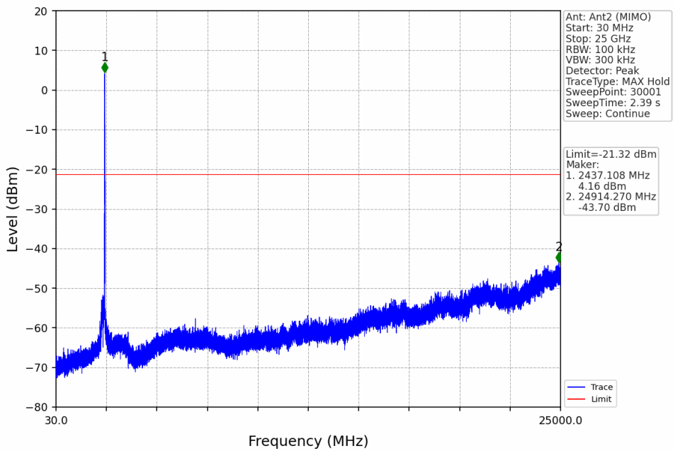
802.11ax(HEW40)_MCH_2437MHz_RU26_Mid_Ant2 (MIMO)_NTNV
