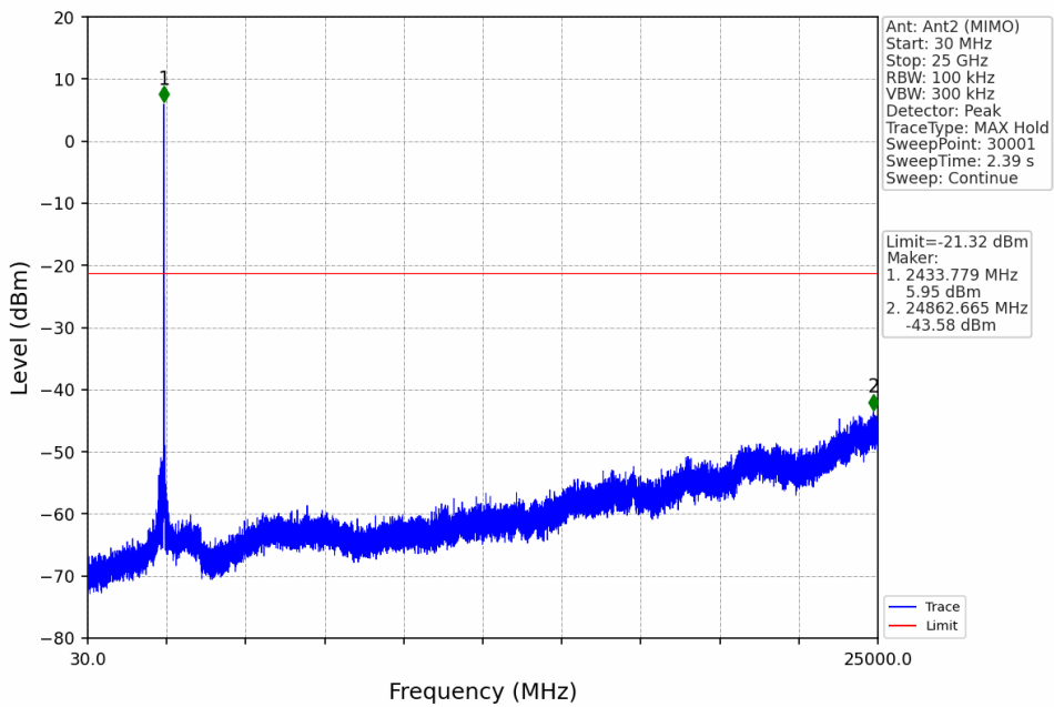
802.11ax(HEW40)_HCH_2452MHz_RU26_Left_Ant2 (MIMO)_NTNV
