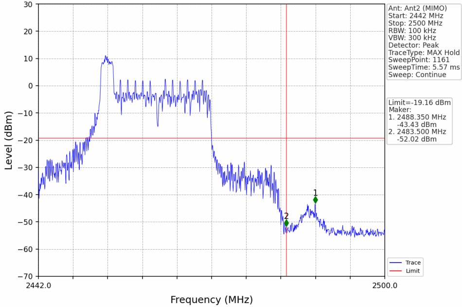
802.11ax(HEW20)_HCH_2462MHz_RU26_Left_Ant2 (MIMO)_NTNV
