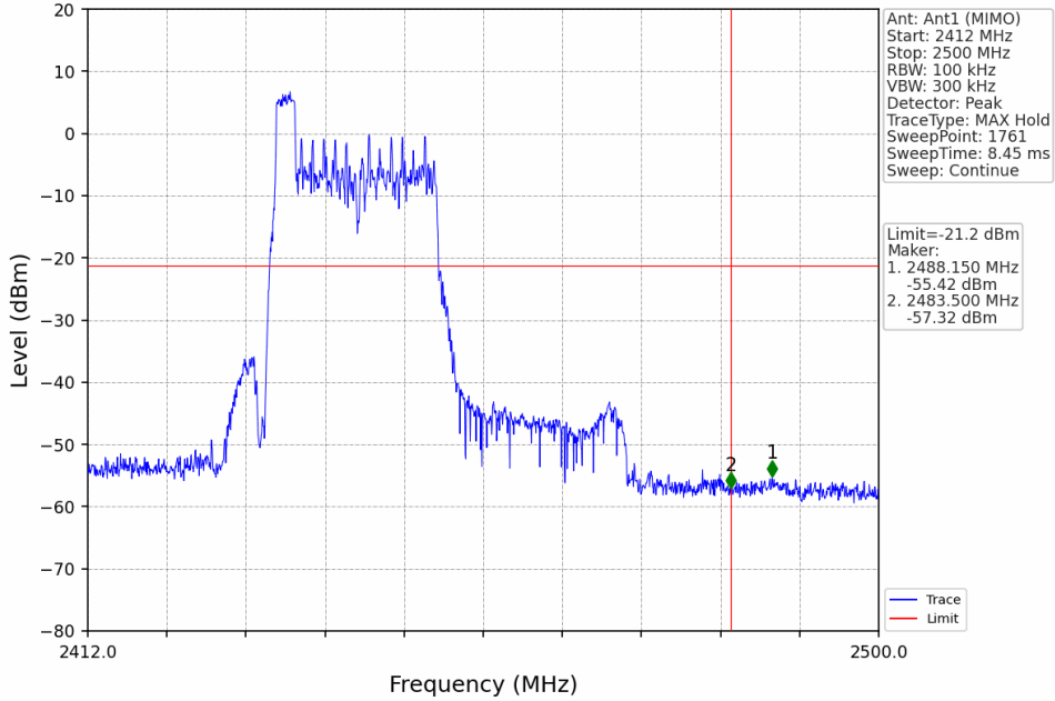
802.11ax(HEW40)_HCH_2452MHz_RU26_Left_Ant1 (MIMO)_NTNV
