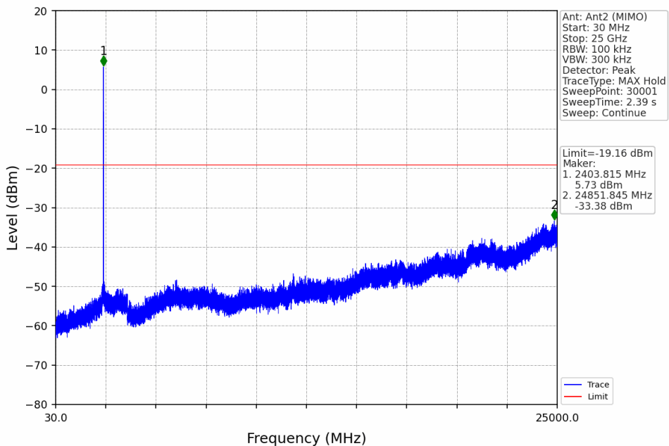
802.11ax(HEW20)_LCH_2412MHz_RU26_Left_Ant2 (MIMO)_NTNV
