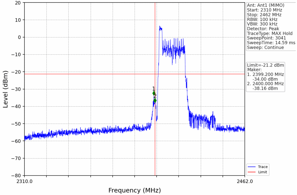
802.11ax(HEW40)_LCH_2422MHz_RU26_Left_Ant1 (MIMO)_NTNV
