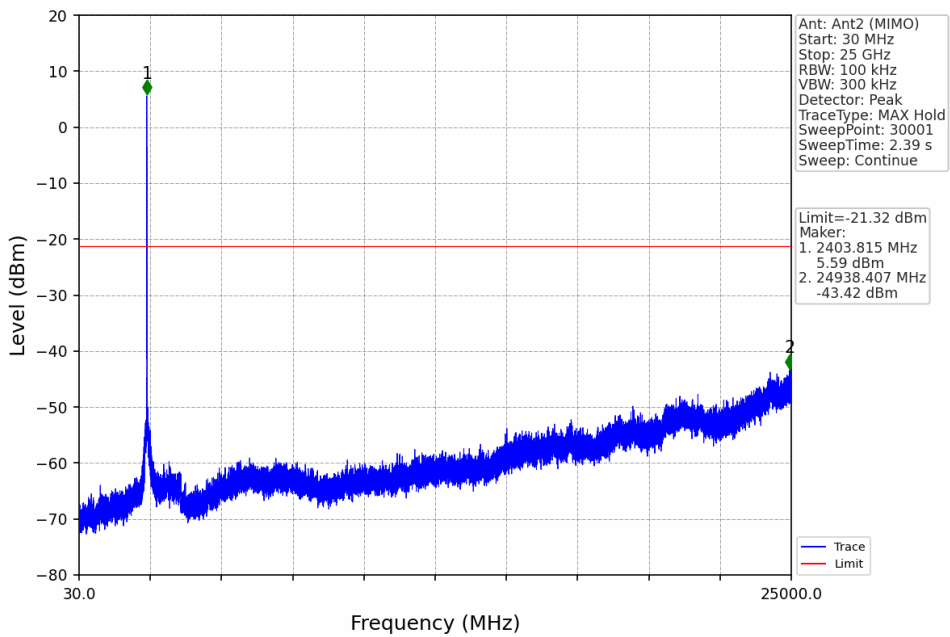
802.11ax(HEW40)_LCH_2422MHz_RU26_Left_Ant2 (MIMO)_NTNV
