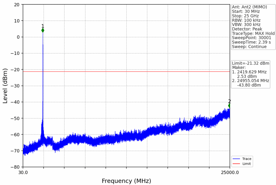
802.11ax(HEW40)_MCH_2437MHz_RU26_Left_Ant2 (MIMO)_NTNV
