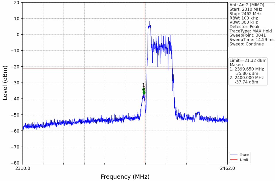
802.11ax(HEW40)_LCH_2422MHz_RU26_Left_Ant2 (MIMO)_NTNV
