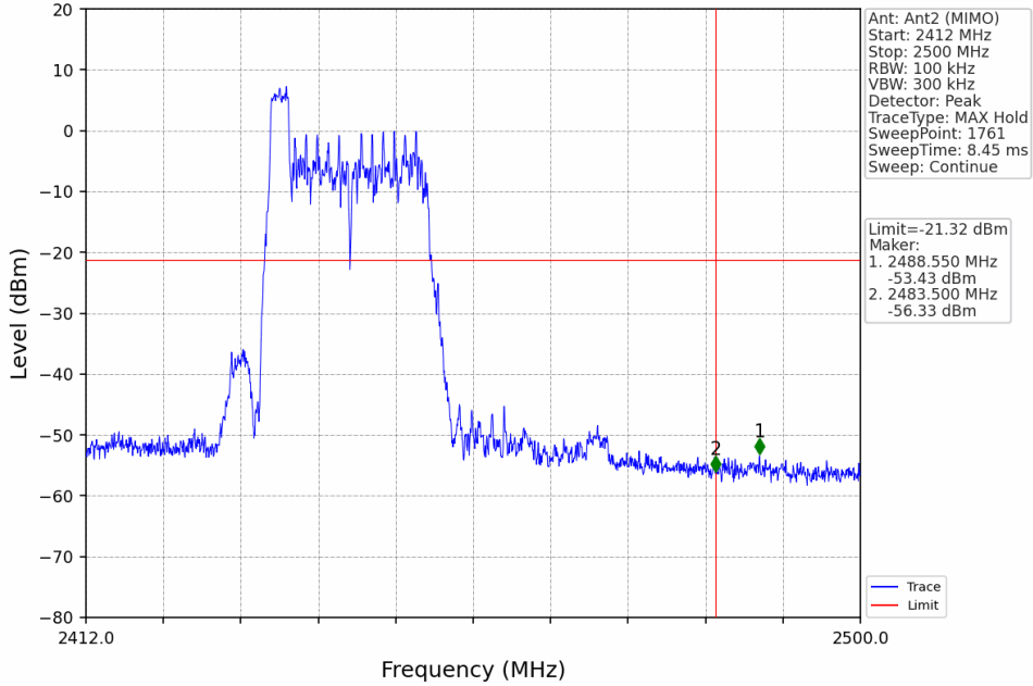
802.11ax(HEW40)_HCH_2452MHz_RU26_Left_Ant2 (MIMO)_NTNV
