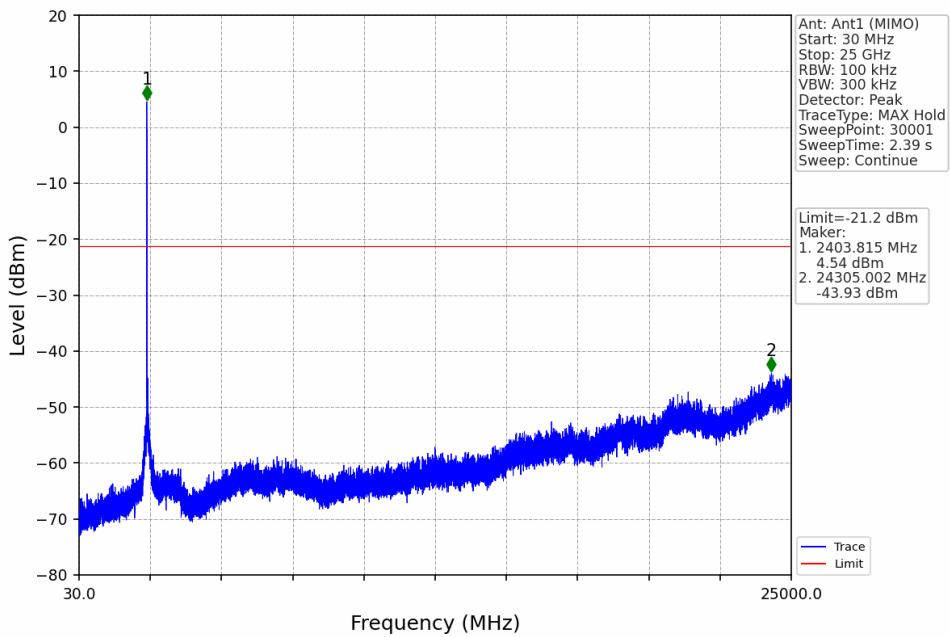
802.11ax(HEW40)_LCH_2422MHz_RU26_Left_Ant1 (MIMO)_NTNV
