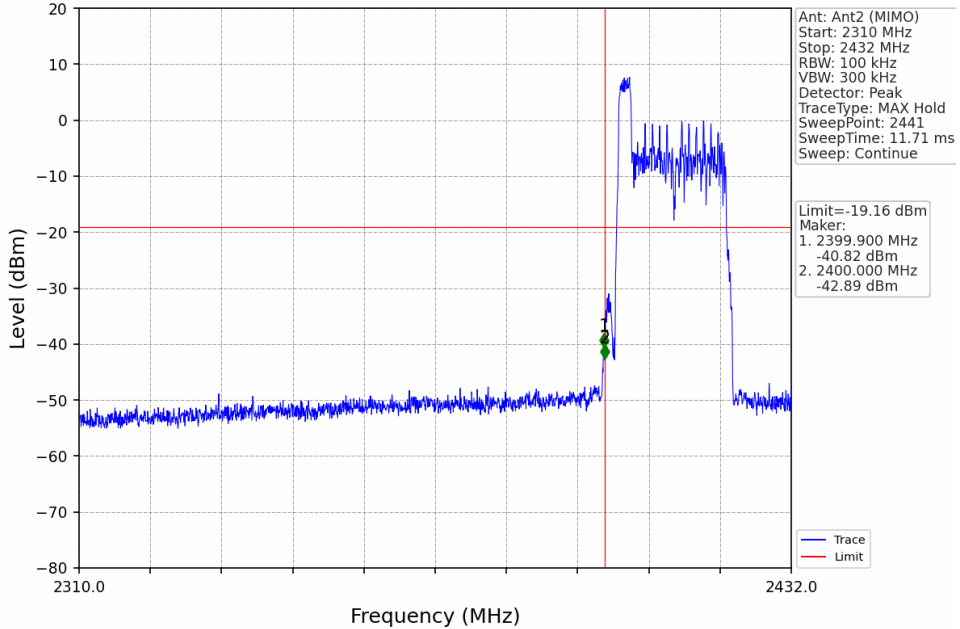
802.11ax(HEW20)_LCH_2412MHz_RU26_Left_Ant2 (MIMO)_NTNV
