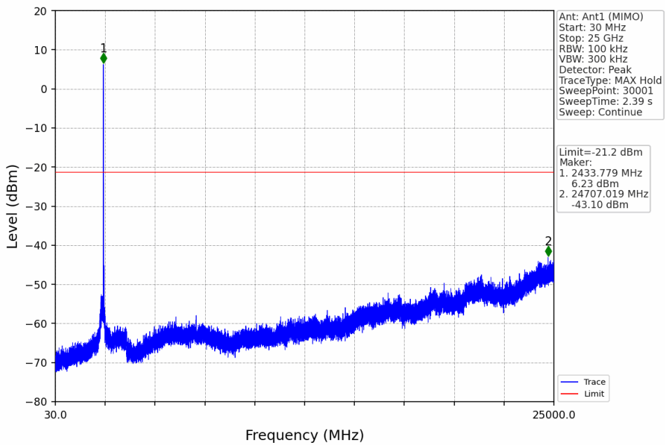
802.11ax(HEW40)_HCH_2452MHz_RU26_Left_Ant1 (MIMO)_NTNV
