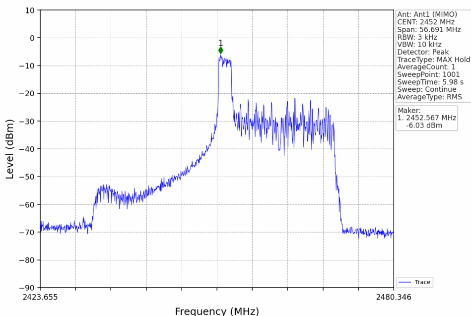
802.11ax(HEW40)_HCH_2452MHz_RU26_Mid_Ant1 (MIMO)_NTNV
