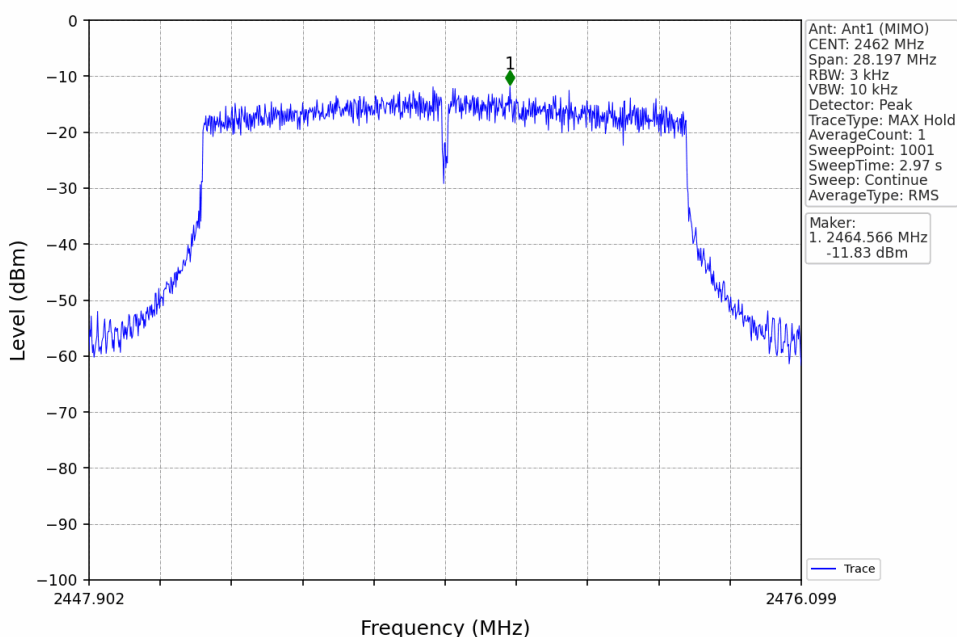
802.11ax(HEW20)_HCH_2462MHz_RU242_Left_Ant1 (MIMO)_NTNV
