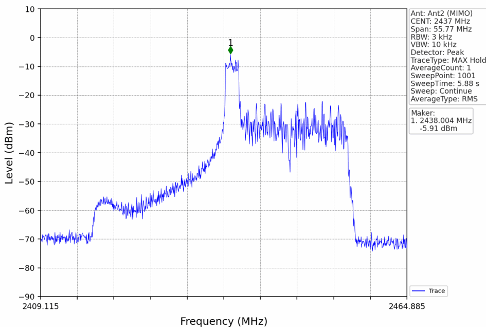
802.11ax(HEW40)_MCH_2437MHz_RU26_Mid_MIMO_NTNV
