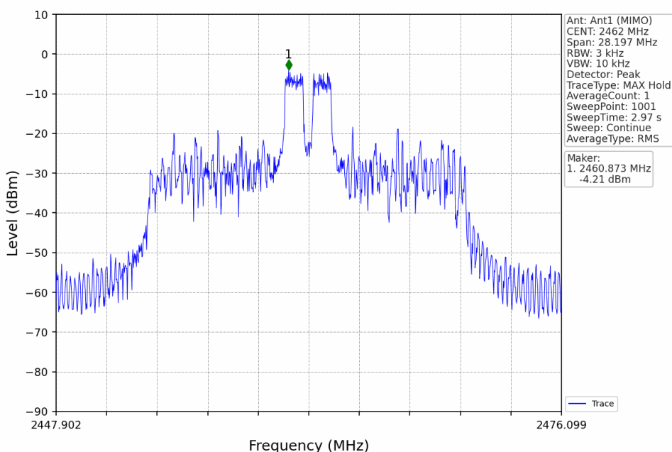
802.11ax(HEW20)_HCH_2462MHz_RU26_Mid_Ant1 (MIMO)_NTNV
