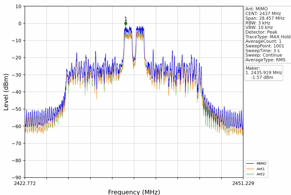
802.11ax(HEW20)_MCH_2437MHz_RU26_Mid_MIMO_NTNV
