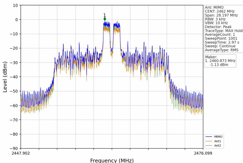
802.11ax(HEW20)_HCH_2462MHz_RU26_Mid_MIMO_NTNV
