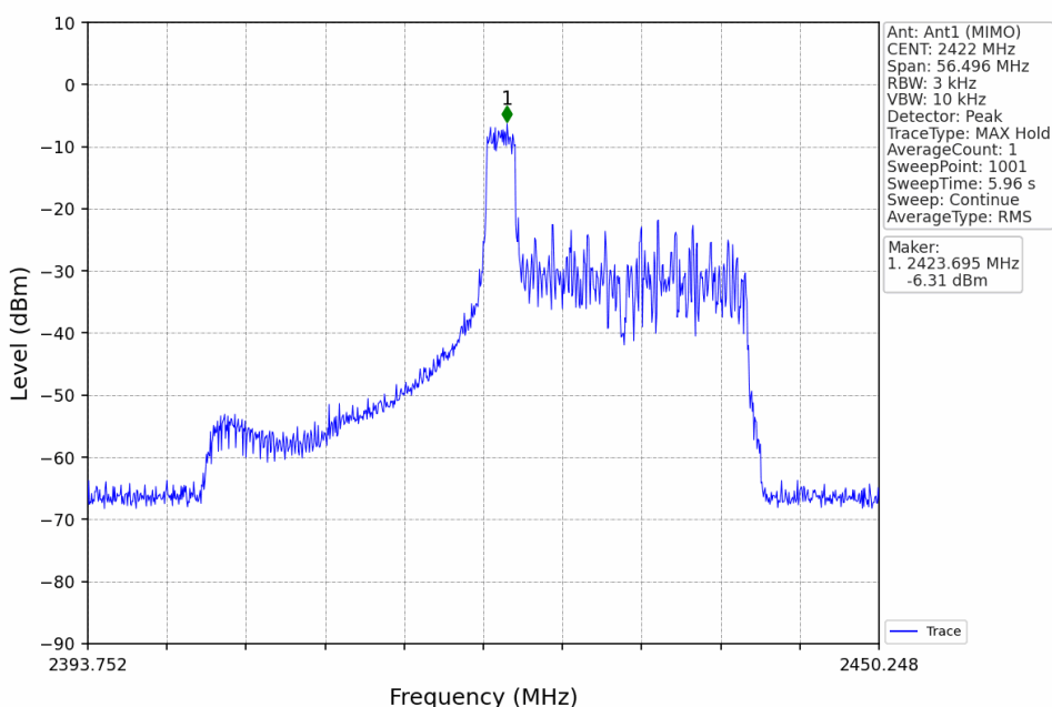
802.11ax(HEW40)_LCH_2422MHz_RU26_Mid_Ant1 (MIMO)_NTNV
