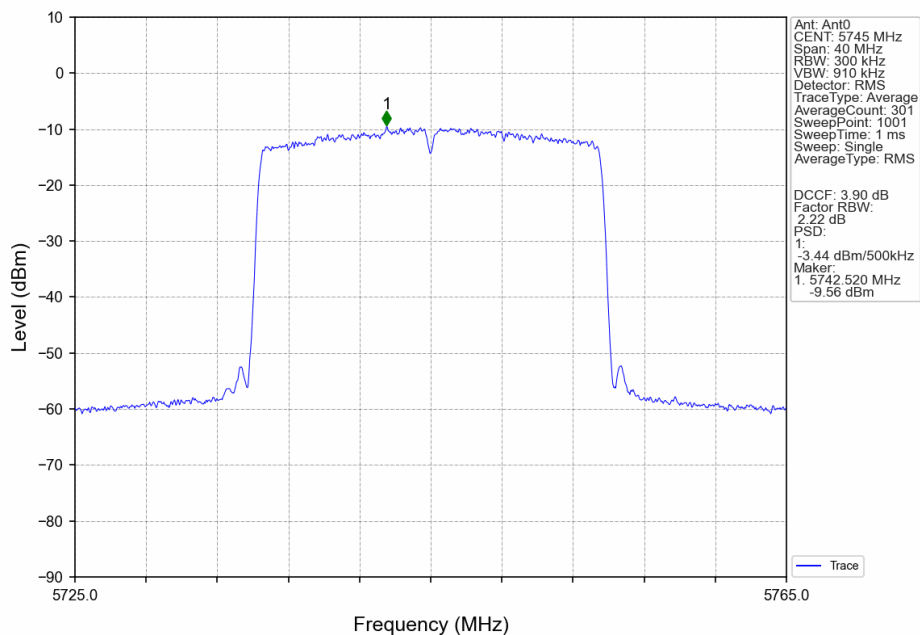
802.11ax(HEW20)_LCH_5745MHz_RU242_Left_Ant0_NTNV
