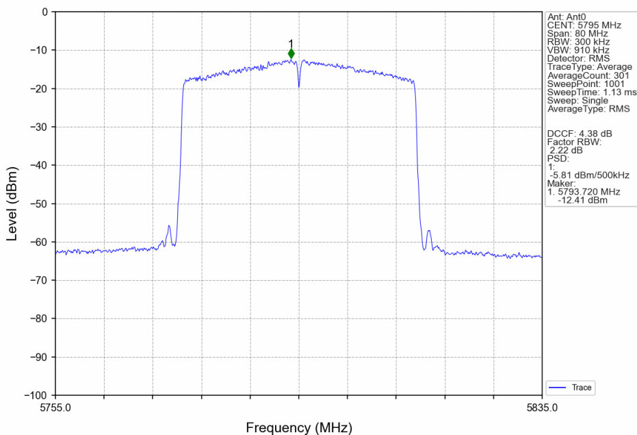
802.11ax(HEW40)_HCH_5795MHz_RU484_Left_Ant0_NTNV
