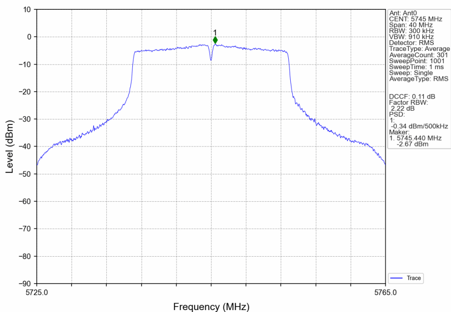
802.11n(HT20)_LCH_5745MHz_Ant0_NTNV
