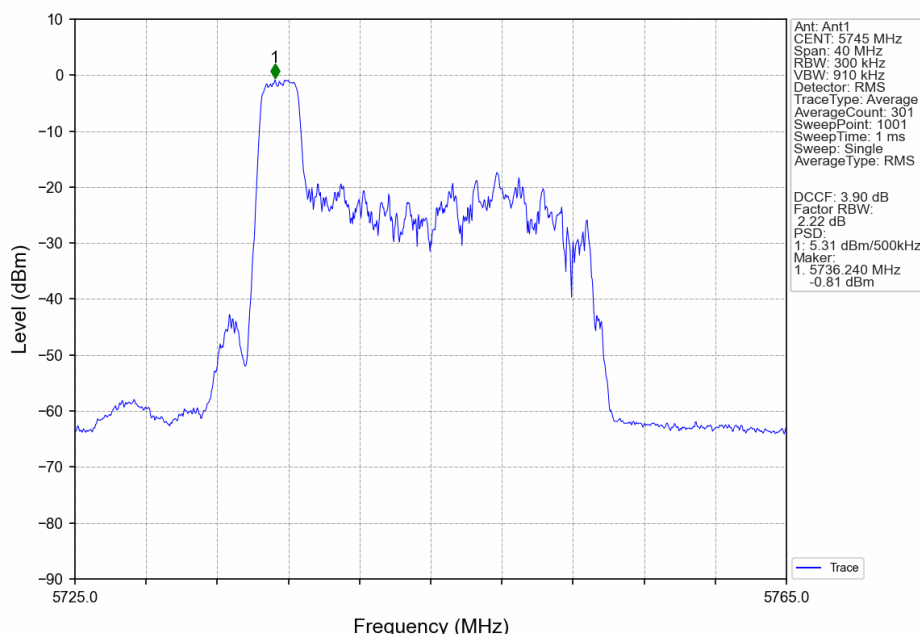
802.11ax(HEW20)_LCH_5745MHz_RU26_Left_Ant1_NTNV
