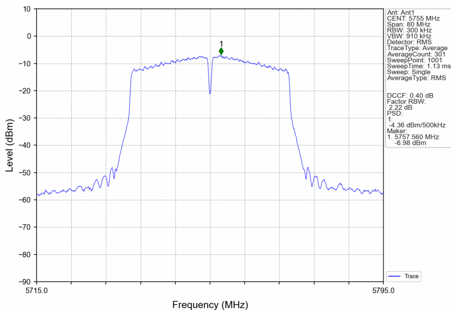
802.11ac(VHT40)_LCH_5755MHz_MIMO_NTNV
