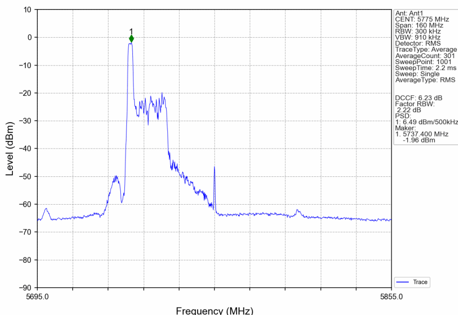
802.11ax(HEW80)_MCH_5775MHz_RU26_Left_Ant1_NTNV
