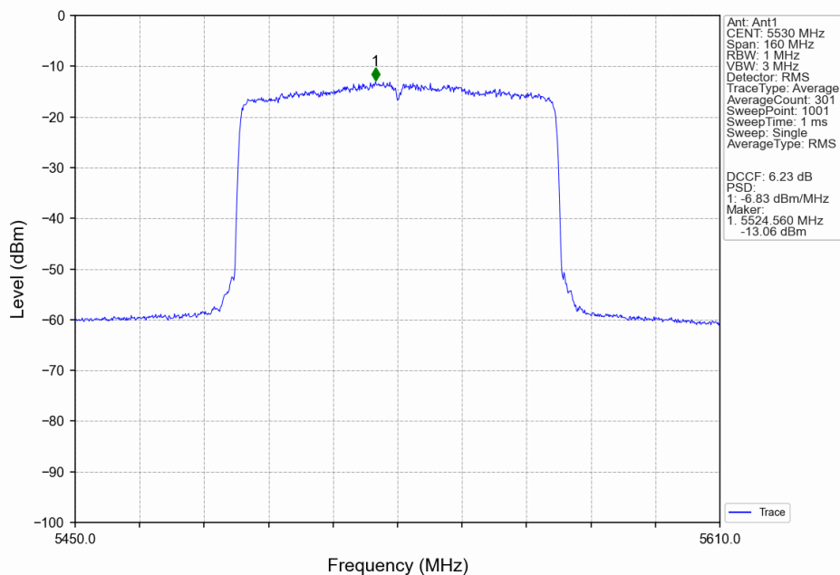
802.11ax(HEW80)_LCH_5530MHz_RU996_Left_Ant1_NTNV
