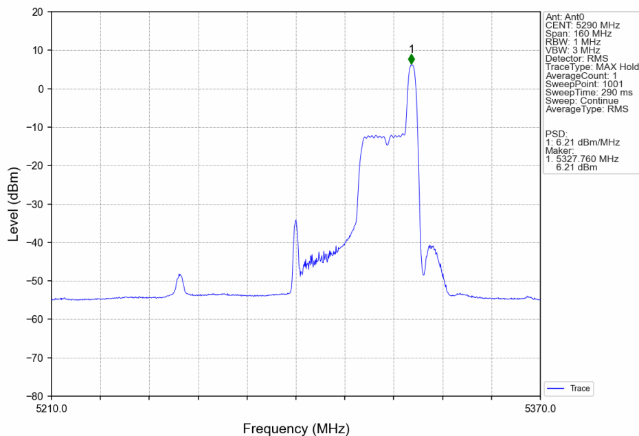
802.11ax(HEW80)_MCH_5290MHz_RU26_Right_Ant0_NTNV
