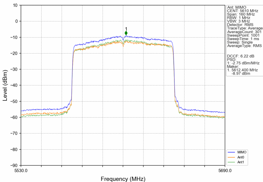
802.11ax(HEW80)_HCH_5610MHz_RU996_Left_MIMO_NTNV
