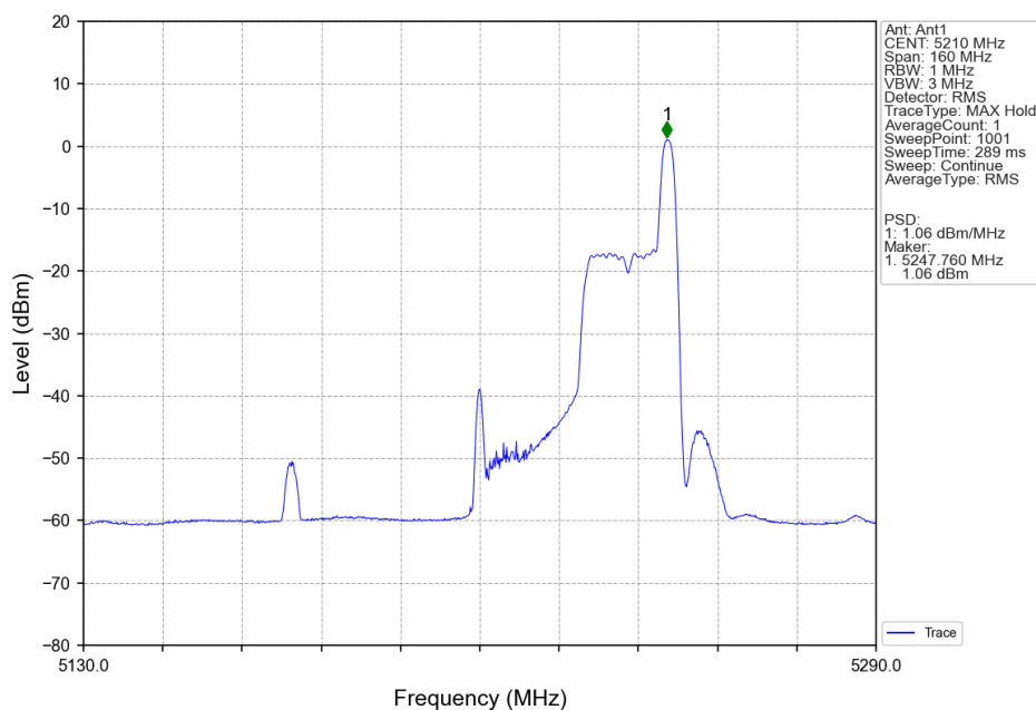
802.11ax(HEW80)_MCH_5210MHz_RU26_Right_Ant1_NTNV
