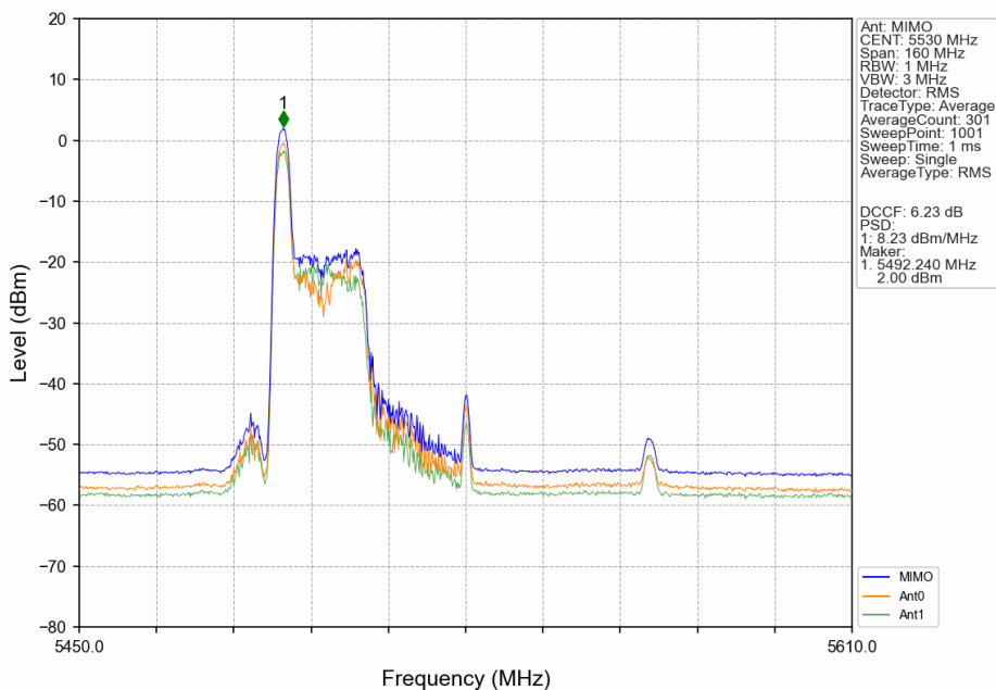
802.11ax(HEW80)_LCH_5530MHz_RU26_Left_MIMO_NTNV
