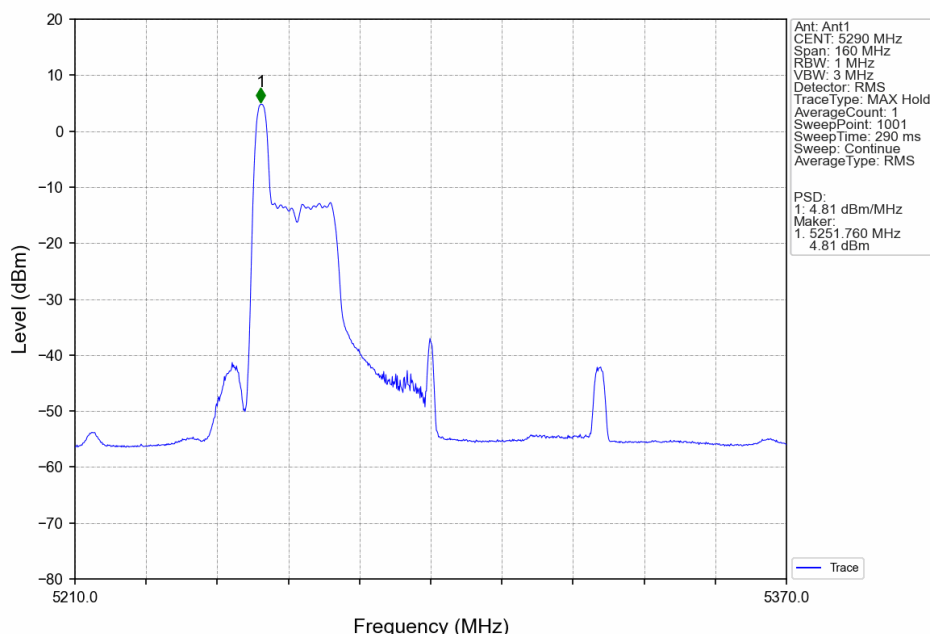
802.11ax(HEW80)_MCH_5290MHz_RU26_Left_Ant1_NTNV
