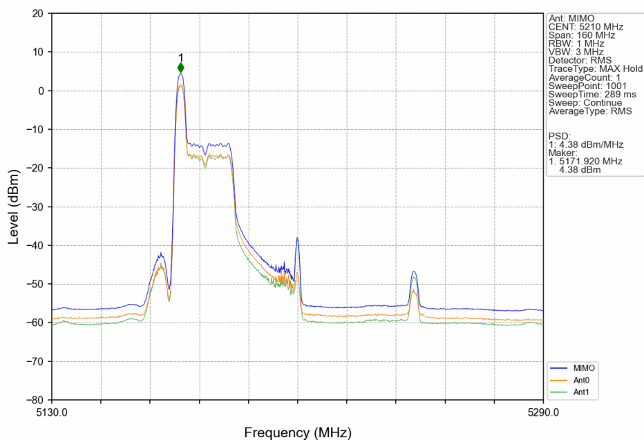
802.11ax(HEW80)_MCH_5210MHz_RU26_Left_MIMO_NTNV
