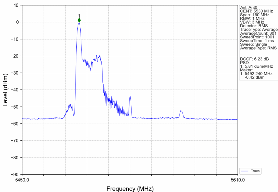
802.11ax(HEW80)_LCH_5530MHz_RU26_Left_Ant0_NTNV
