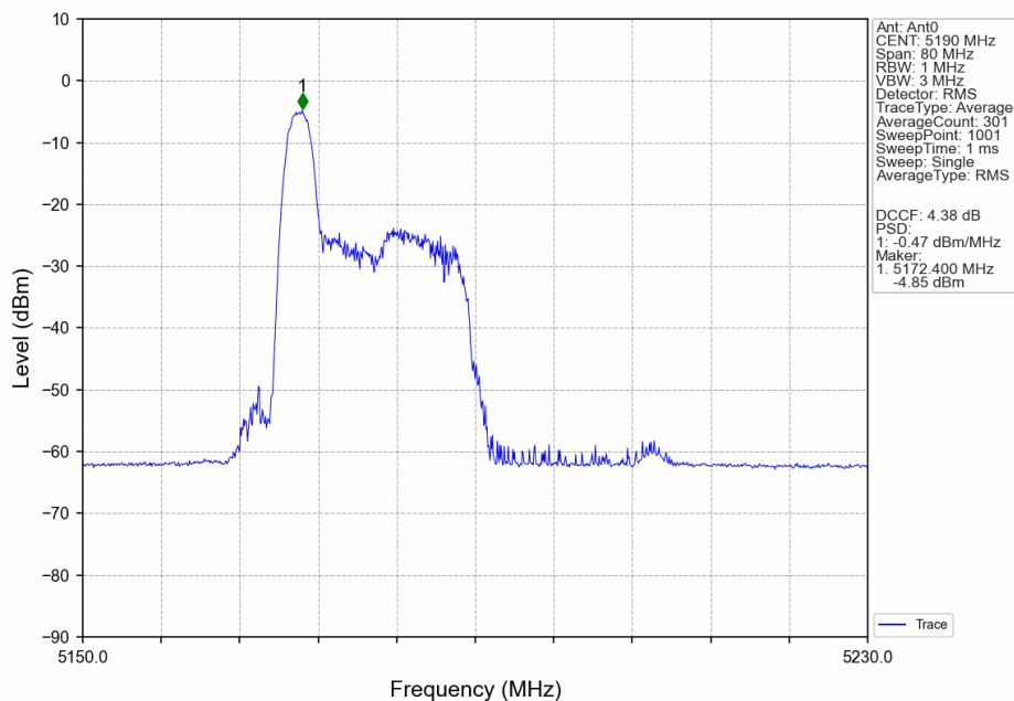
802.11ax(HEW40)_LCH_5190MHz_RU26_Left_Ant0_NTNV
