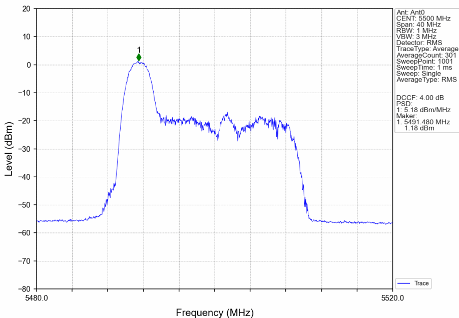
802.11ax(HEW20)_LCH_5500MHz_RU26_Left_Ant0_NTNV
