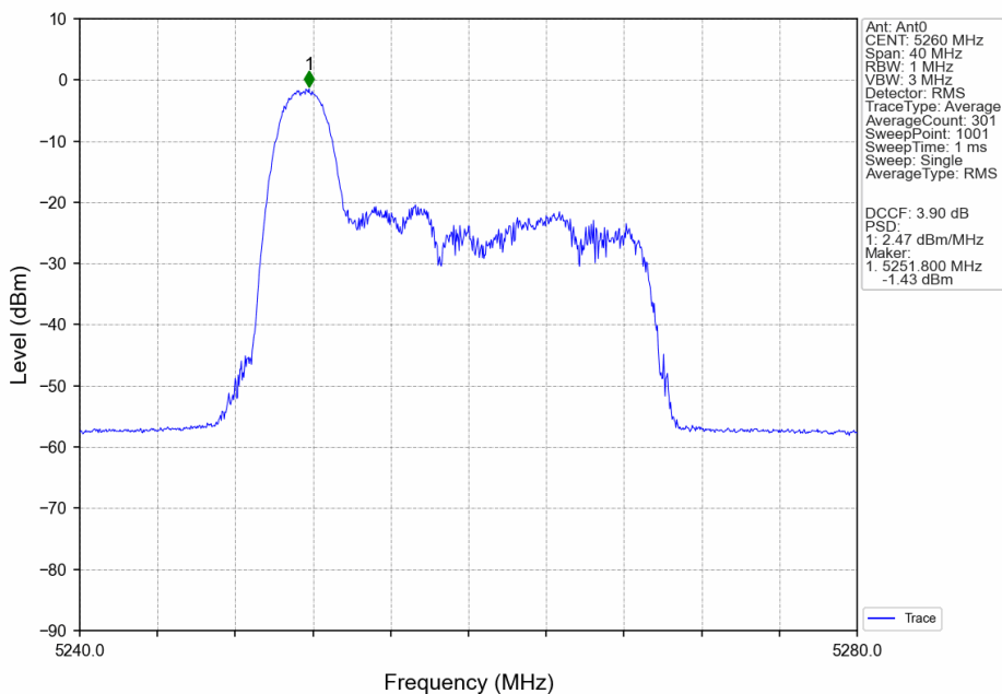
802.11ax(HEW20)_LCH_5260MHz_RU26_Left_Ant0_NTNV
