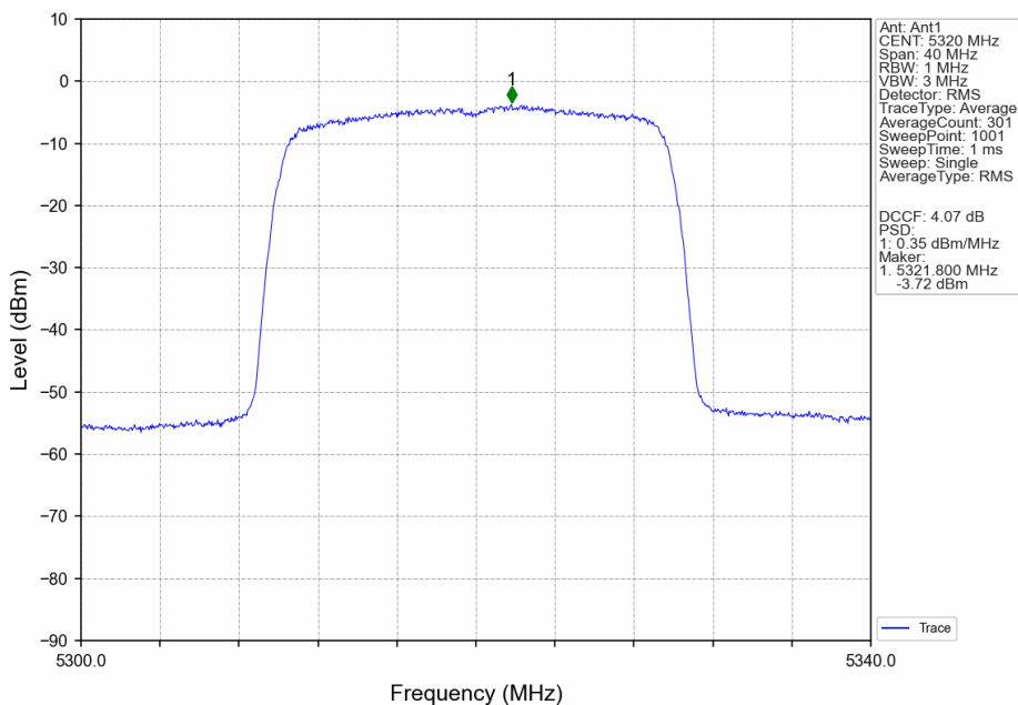
802.11ax(HEW20)_HCH_5320MHz_RU242_Left_Ant1_NTNV
