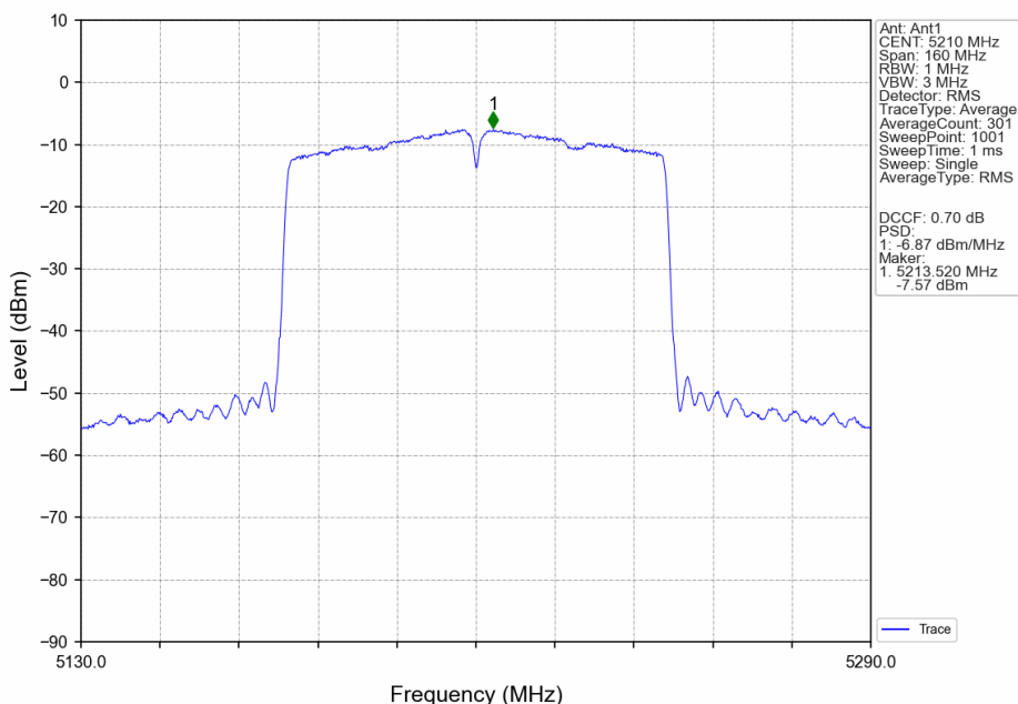
802.11ac(VHT80)_MCH_5210MHz_MIMO_NTNV
