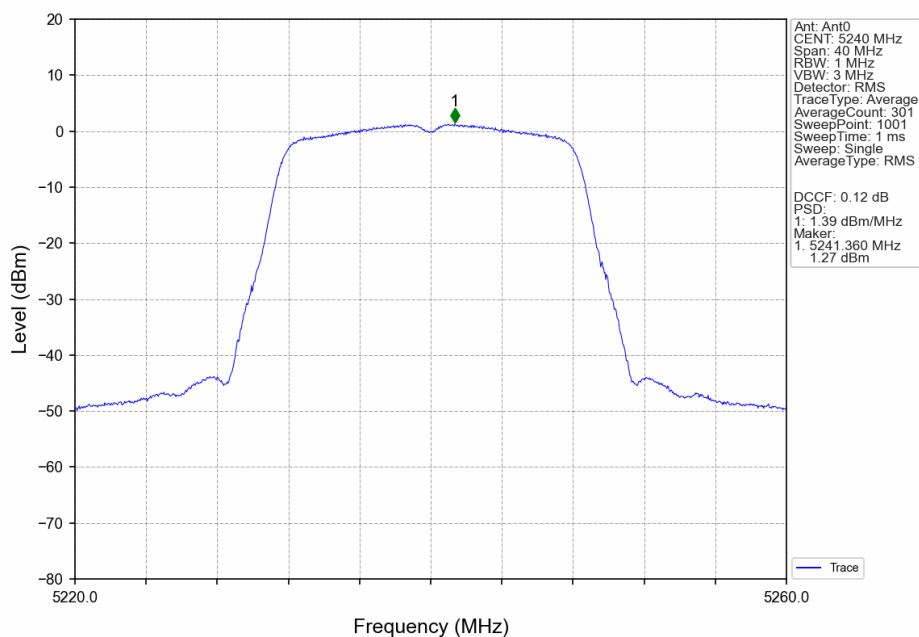
802.11n(HT20)_HCH_5240MHz_Ant0_NTNV
