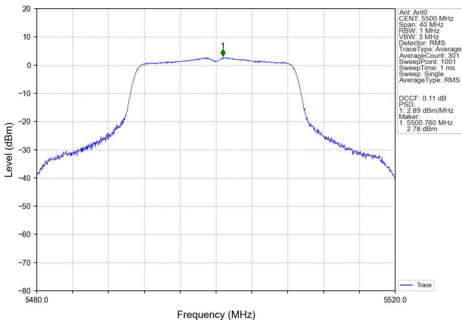
802.11n(HT20)_LCH_5500MHz_Ant0_NTNV
