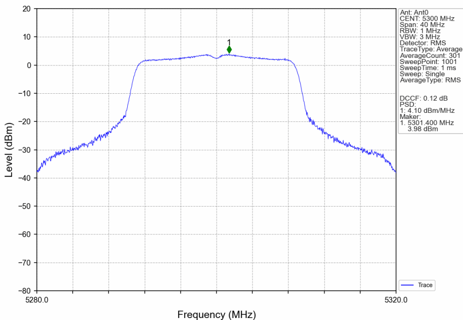
802.11n(HT20)_MCH_5300MHz_Ant0_NTNV
