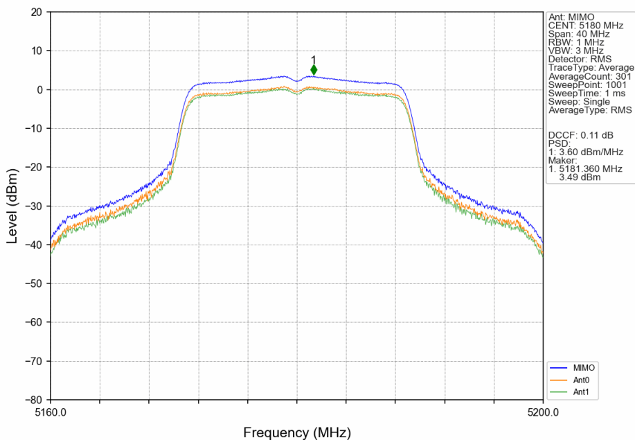
802.11n(HT20)_LCH_5180MHz_MIMO_NTNV
