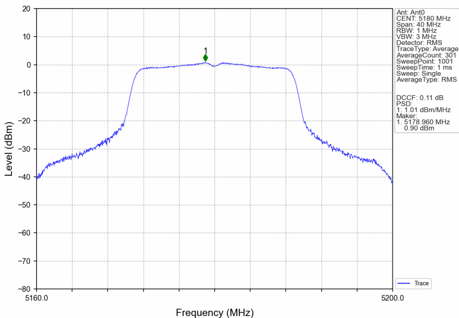
802.11n(HT20)_LCH_5180MHz_Ant0_NTNV
