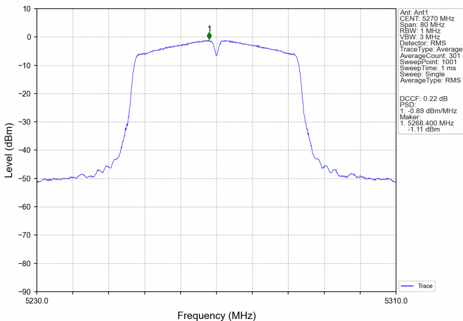
802.11n(HT40)_LCH_5270MHz_Ant1_NTNV
