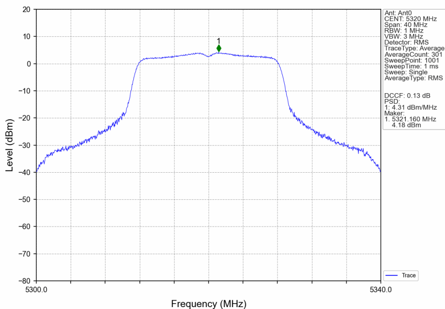
802.11a_HCH_5320MHz_Ant0_NTNV
