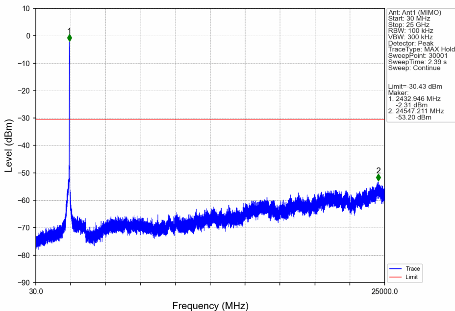
802.11n(HT40)_MCH_2437MHz_Ant1 (MIMO)_NTNV
