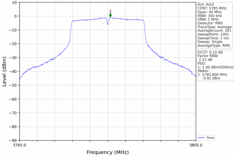
802.11a_MCH_5785MHz_MIMO_NTNV
