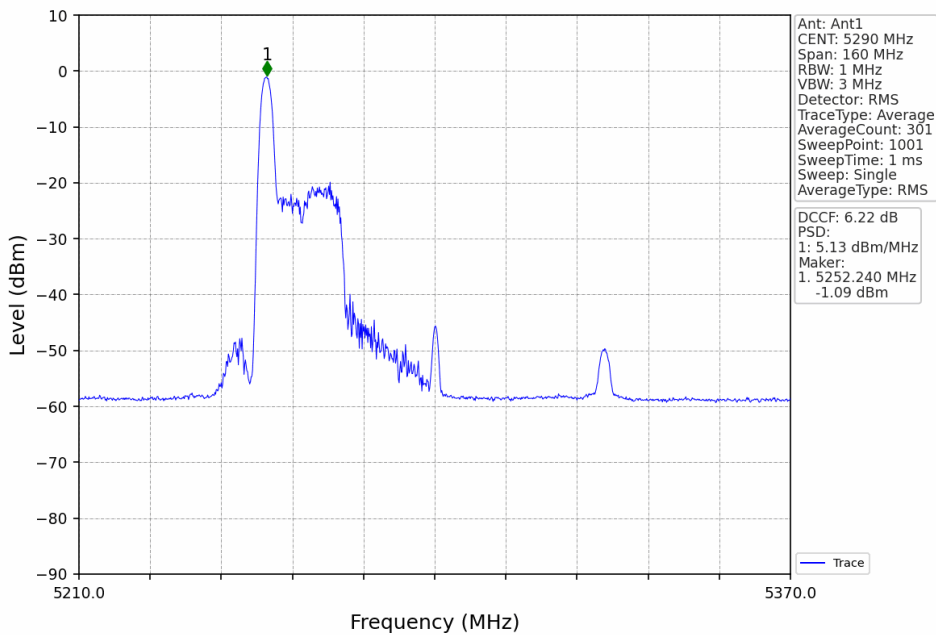
802.11ax(HEW80)_MCH_5290MHz_RU26_Left_Ant1_NTNV
