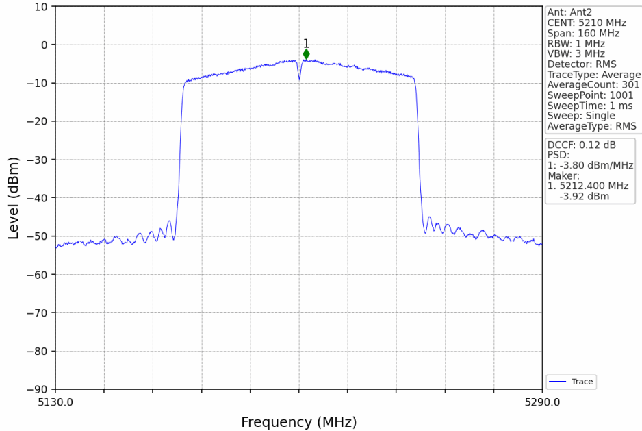
802.11ac(VHT80)_MCH_5210MHz_MIMO_NTNV
