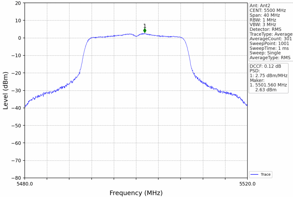
802.11n(HT20)_LCH_5500MHz_MIMO_NTNV
