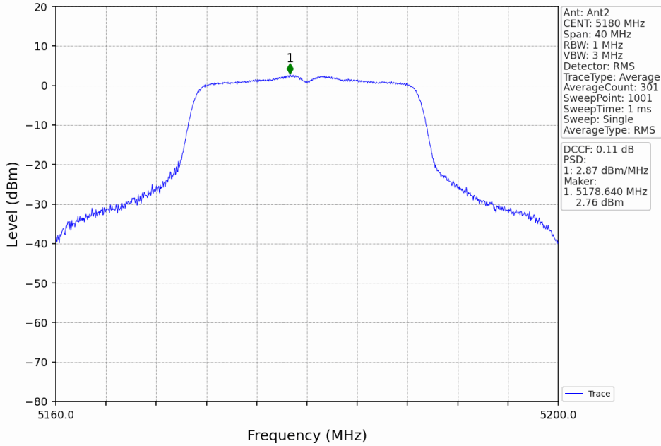
802.11n(HT20)_LCH_5180MHz_MIMO_NTNV
