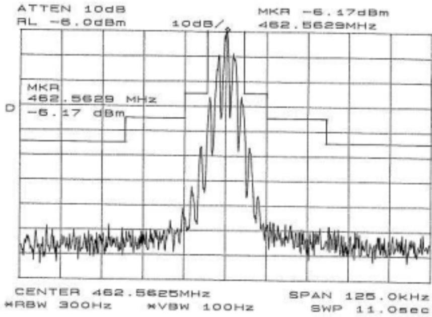
GMRS+CTCSS(167.9Hz)
