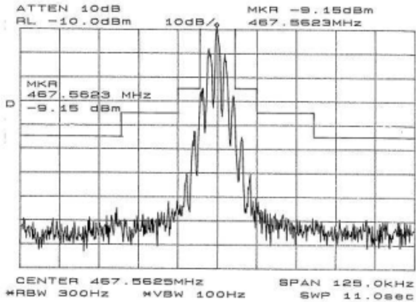
FRS+CTCSS(167.9Hz)
