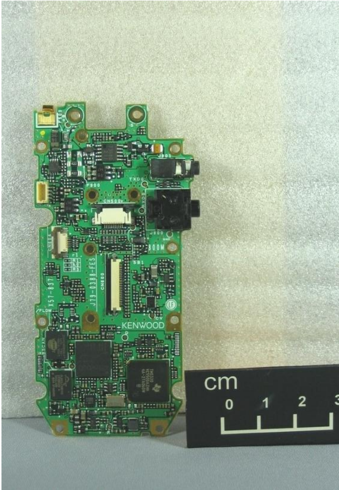
NX-420-K, NX-420-K3 TXRX Unit
