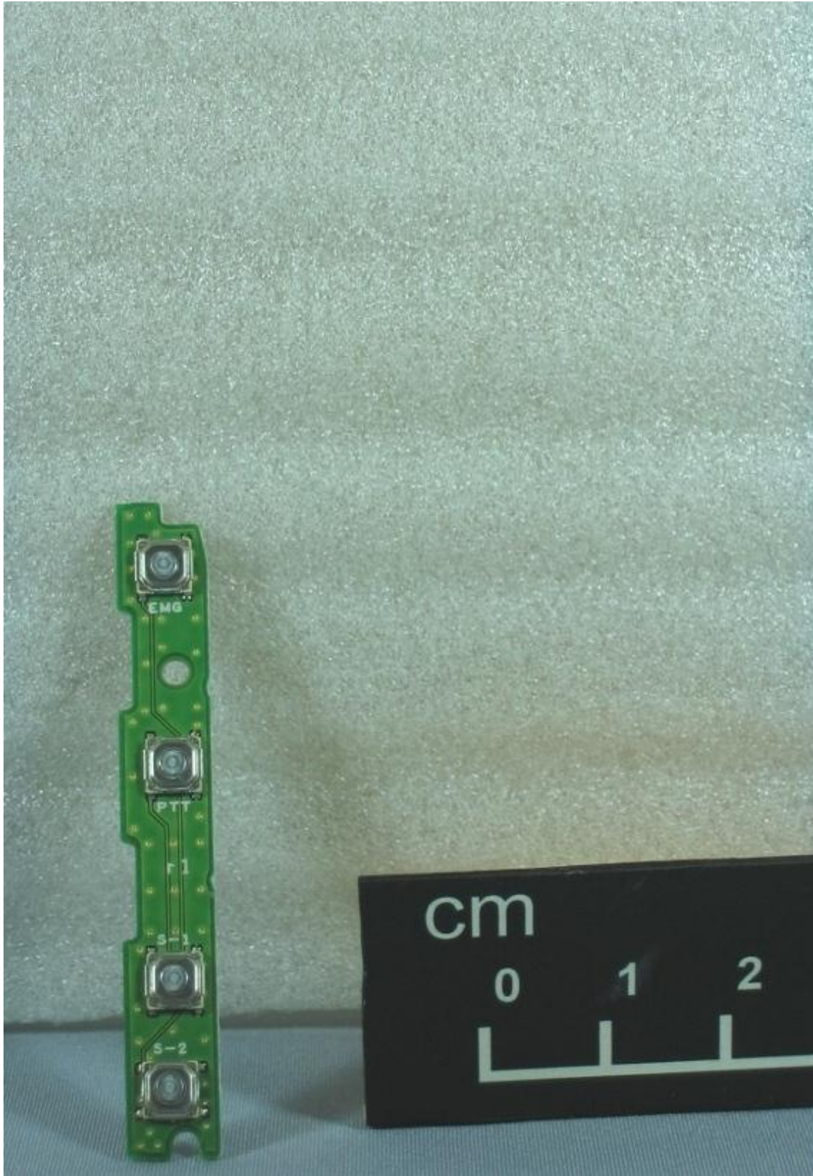
NX-420-K, NX-420-K3 Key
