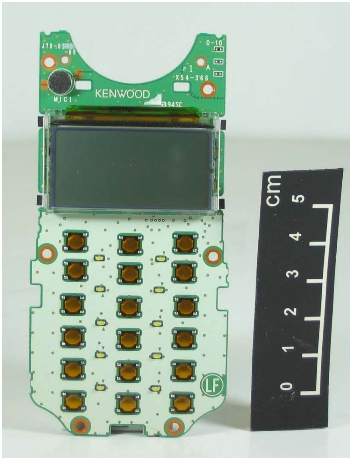
DISPLAY UNIT
