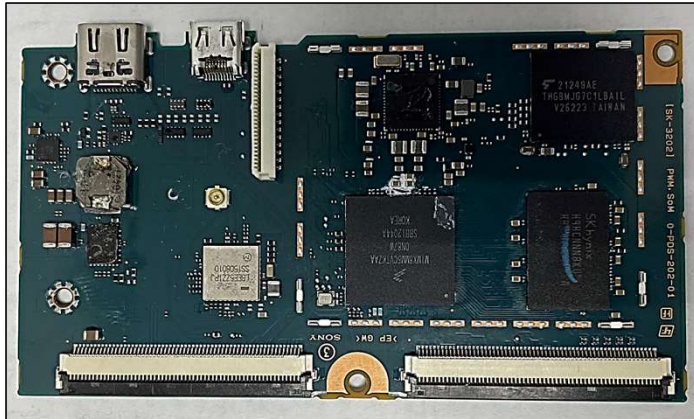
SOM PWB ( Front Side )
