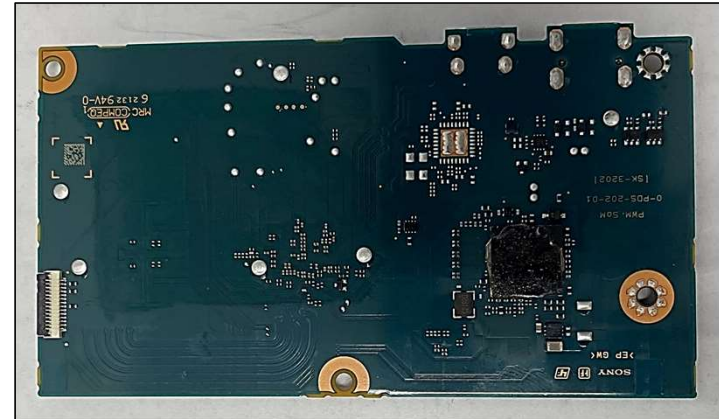
SOM PWB ( Back Side )
