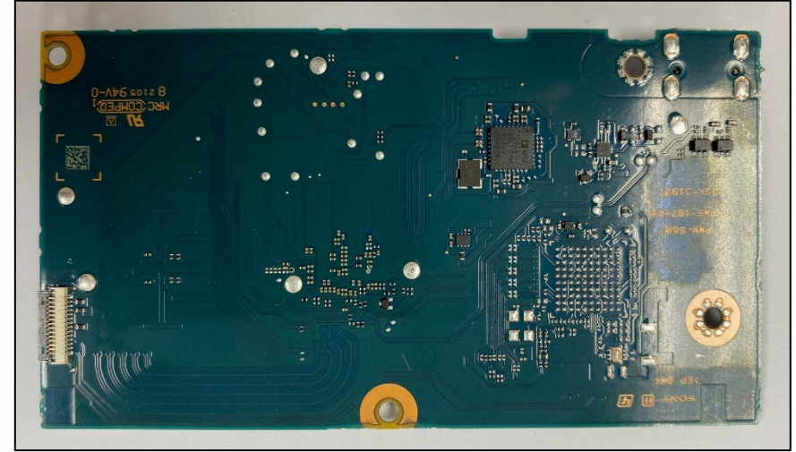
SOM PWB ( Back Side )
