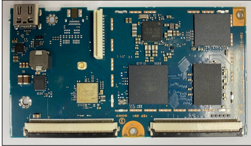
SOM PWB ( Front Side )
