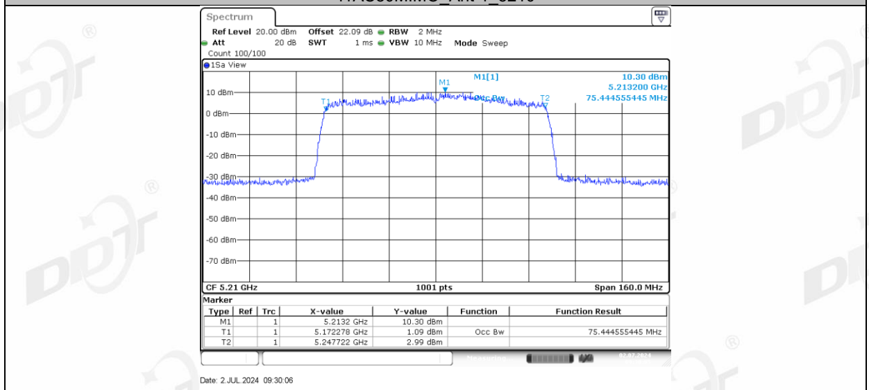
11AC80MIMO_Ant-3_5210
