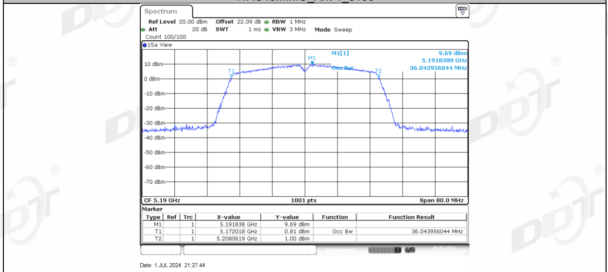
11AC40MIMO_Ant-3_5190
