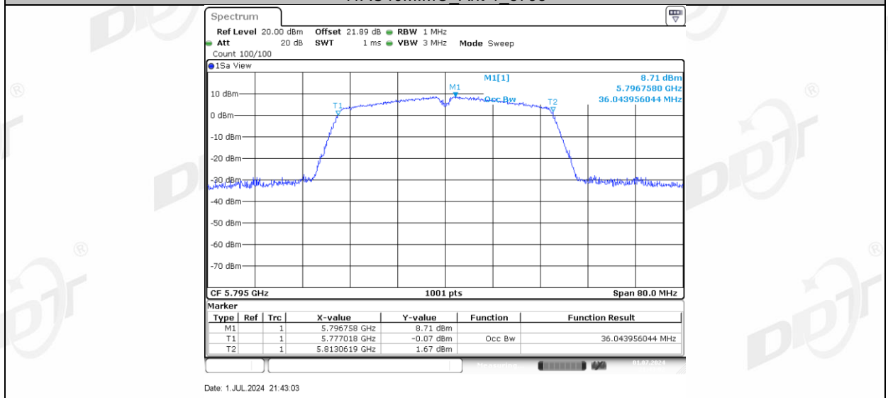
11AC40MIMO_Ant-3_5795
