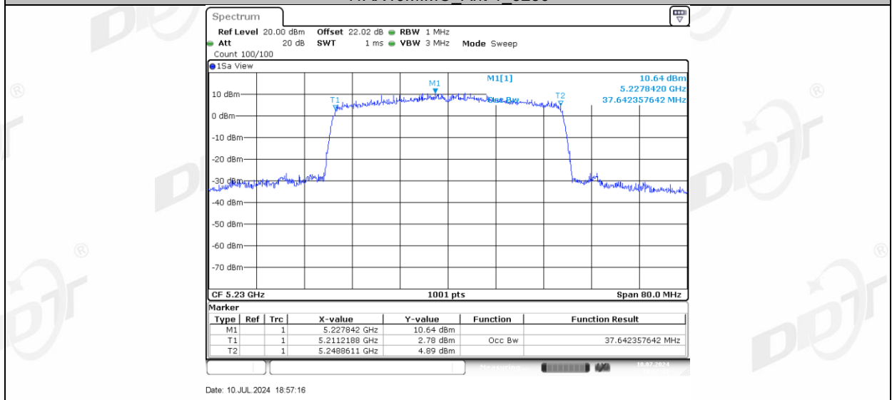
11AX40MIMO_Ant-3_5230
