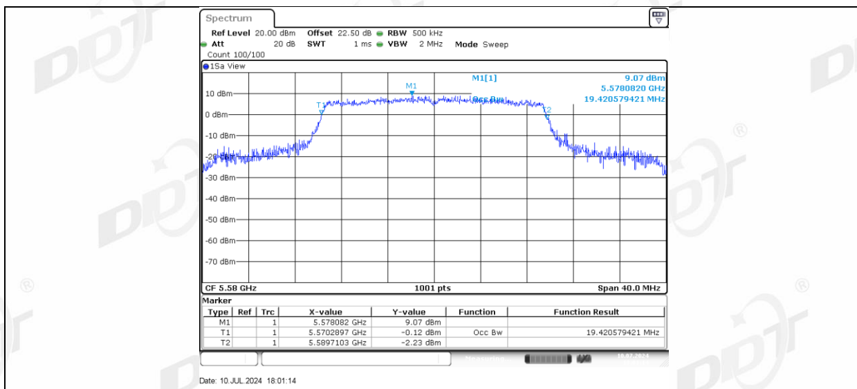
11AX20MIMO_Ant-3_5580
