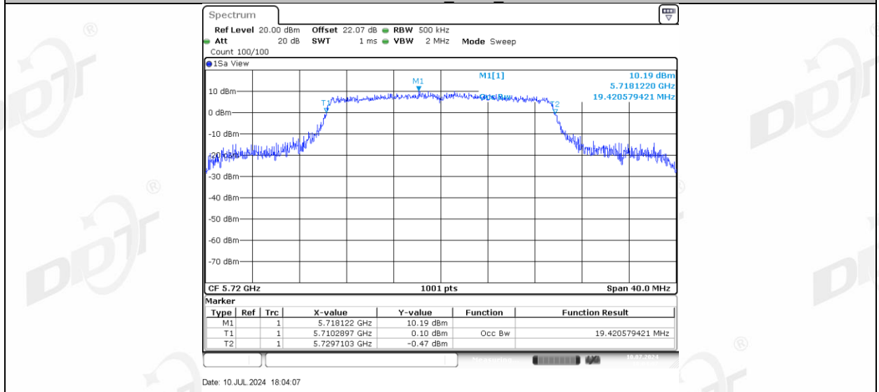
11AX20MIMO_Ant-3_5720
