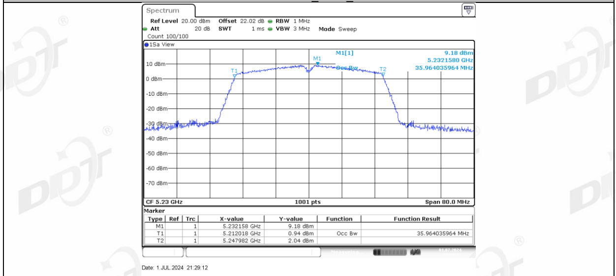
11AC40MIMO_Ant-3_5230
