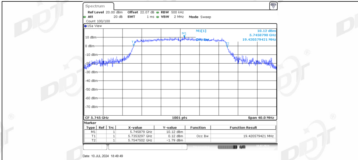
11AX20MIMO_Ant-3_5745
