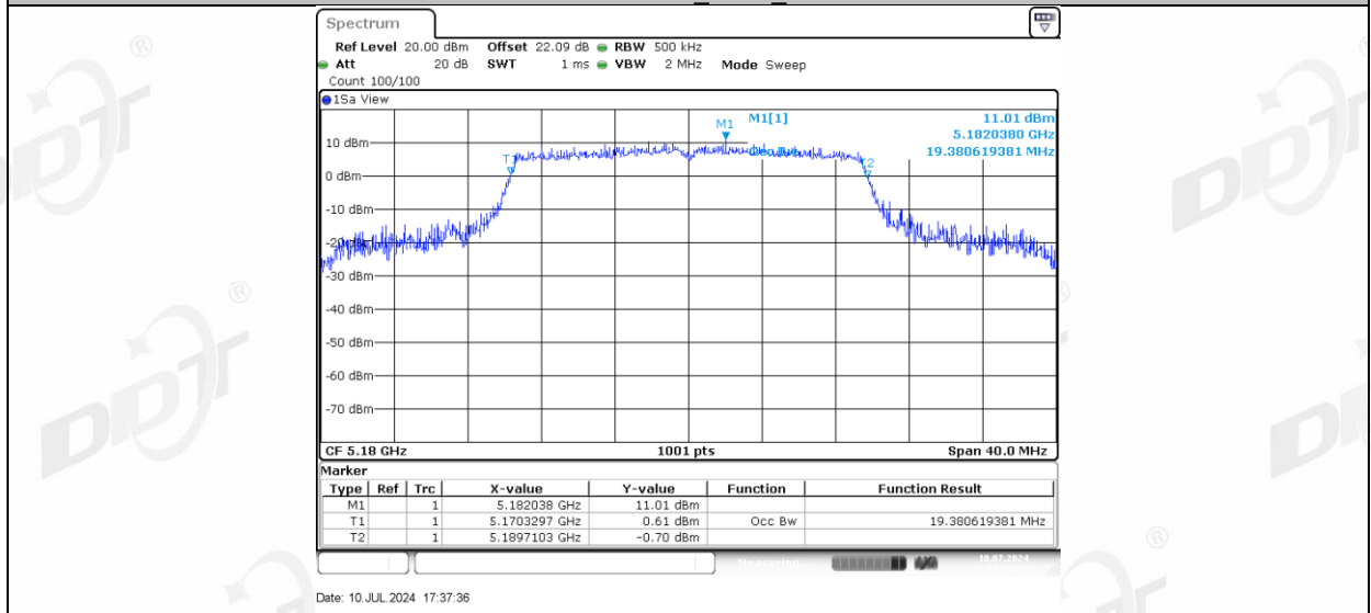
11AX20MIMO_Ant-3_5180
