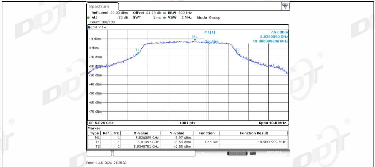
11AC20MIMO_Ant-3_5825
