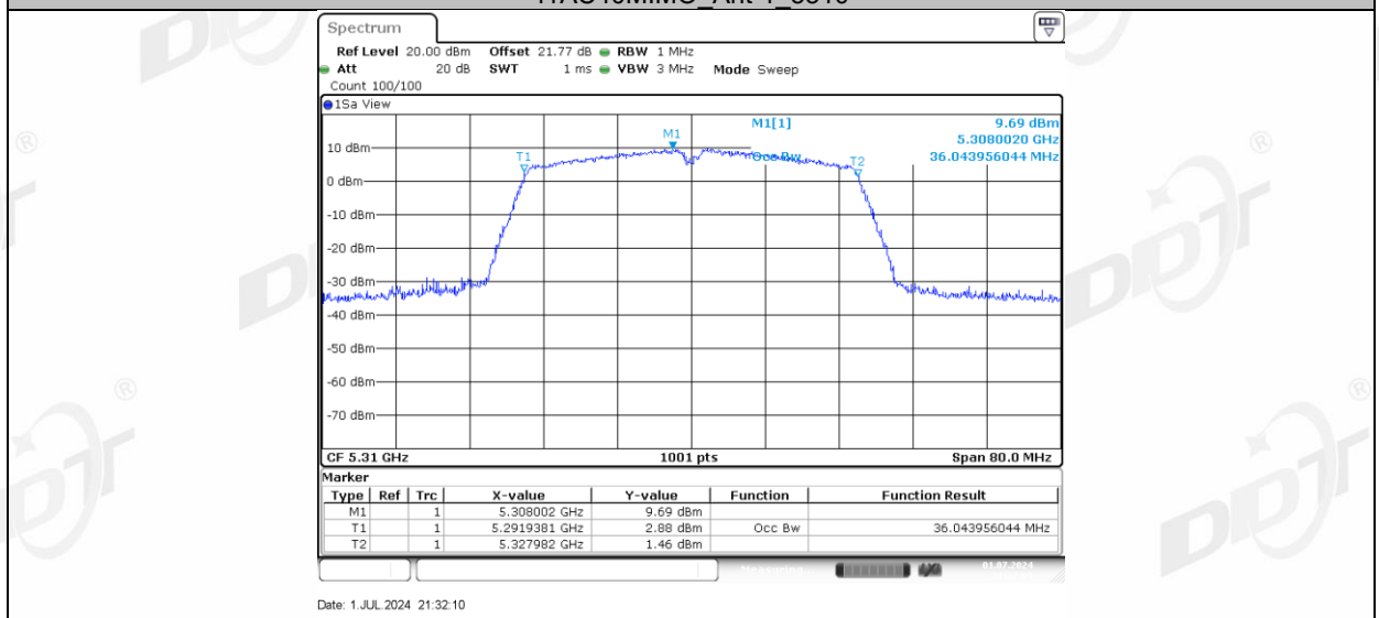
11AC40MIMO_Ant-3_5310
