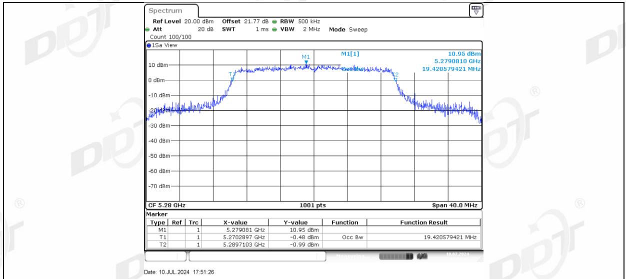
11AX20MIMO_Ant-3_5280
