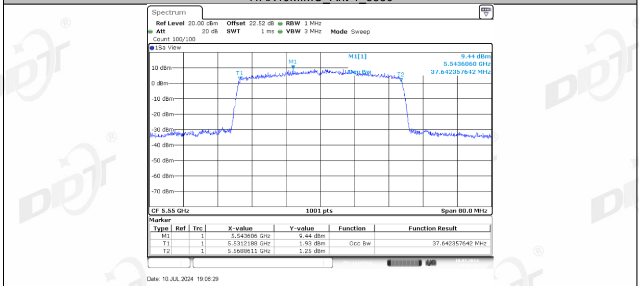
11AX40MIMO Ant-3 5550
