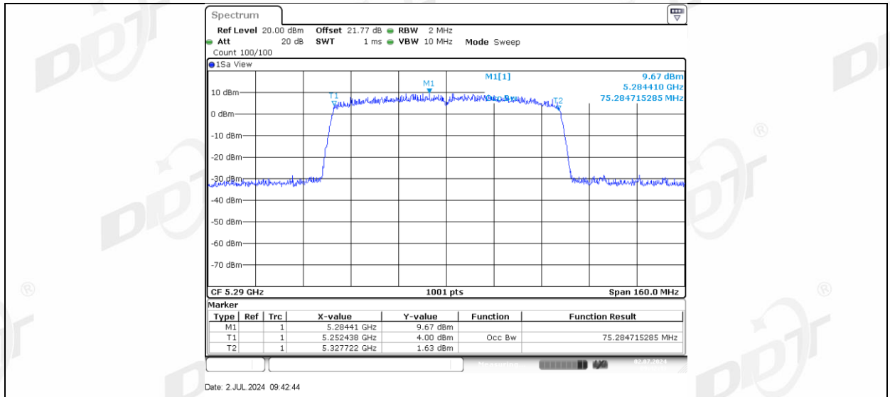
11AC80MIMO_Ant-3_5290
