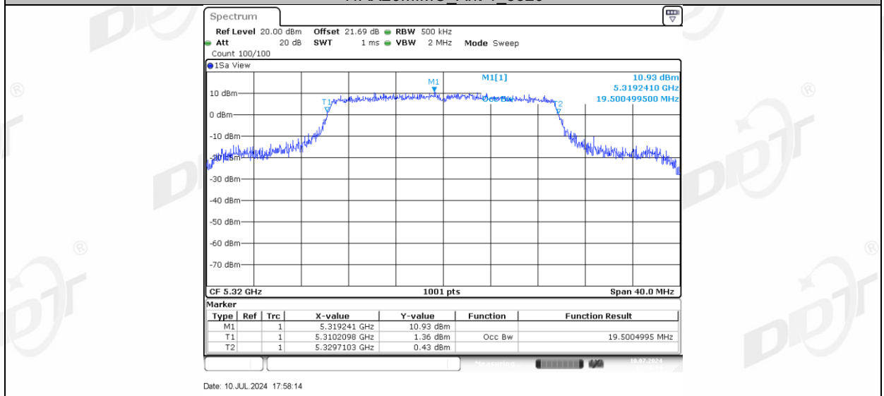
11AX20MIMO_Ant-3_5320
