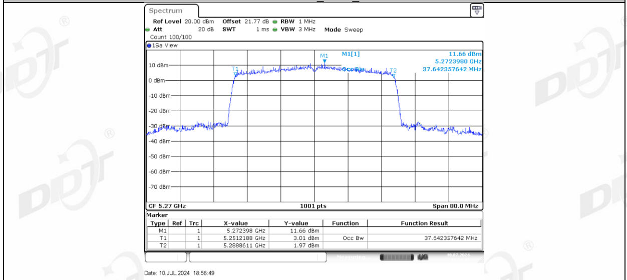
11AX40MIMO Ant-3 5270
