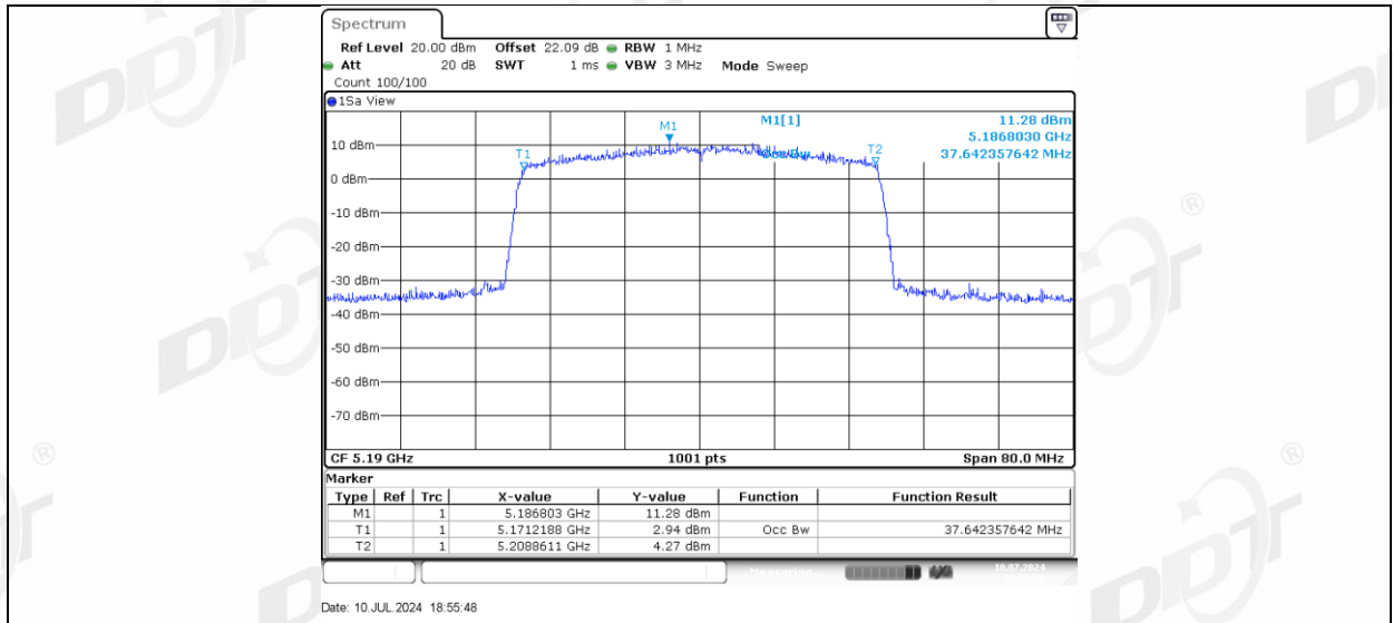
11AX40MIMO_Ant-3_5190
