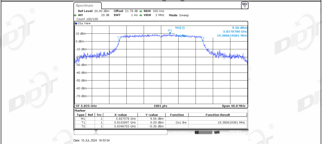
11AX20MIMO_Ant-3_5825
