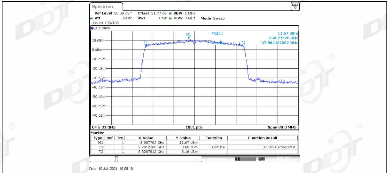
11AX40MIMO_Ant-3_5310
