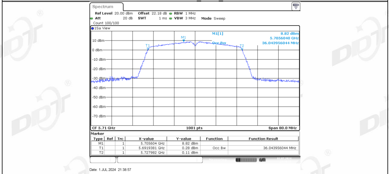
11AC40MIMO_Ant-3_5710
