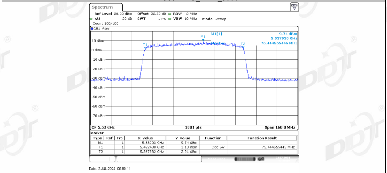
11AC80MIMO_Ant-3_5530
