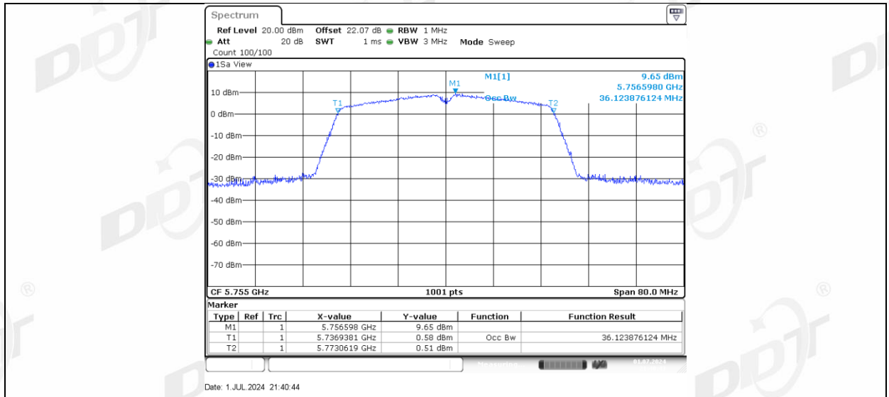
11AC40MIMO_Ant-3_5755
