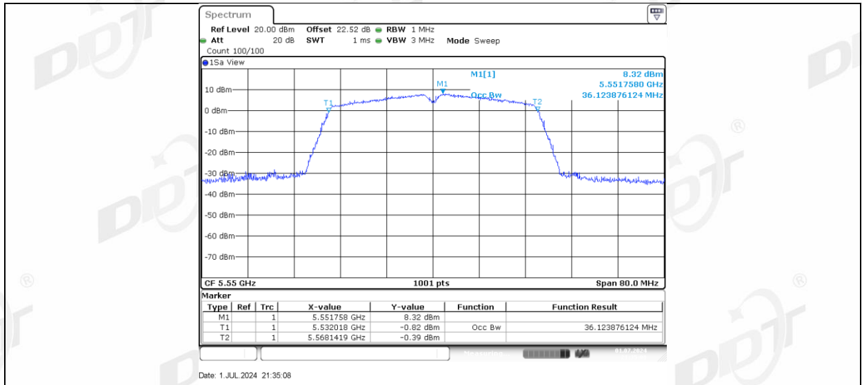
11AC40MIMO_Ant-3_5550
