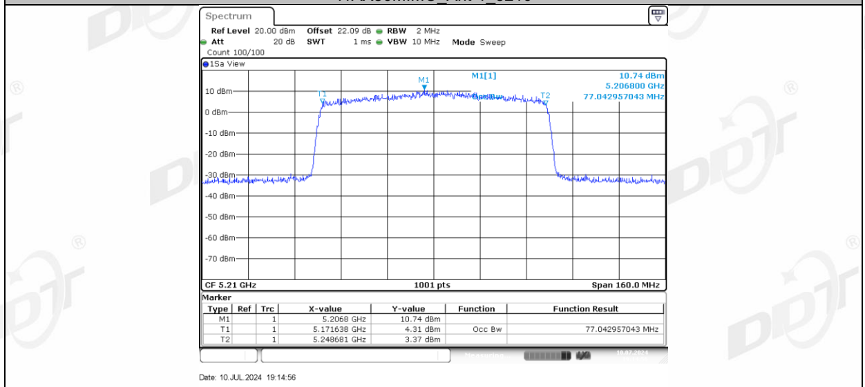
11AX80MIMO_Ant-3_5210
