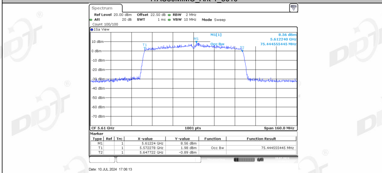
11AC80MIMO_Ant-3_5610
