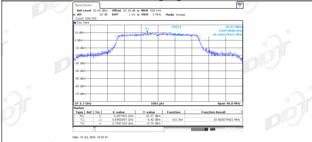
11AX20MIMO_Ant-3_5700
