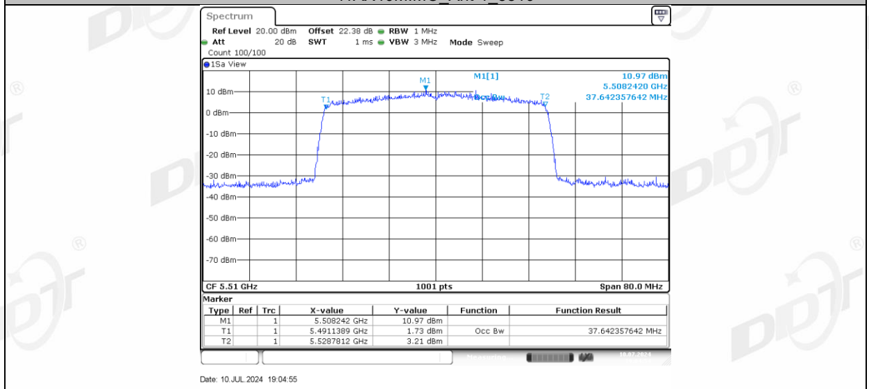
11AX40MIMO_Ant-3_5510
