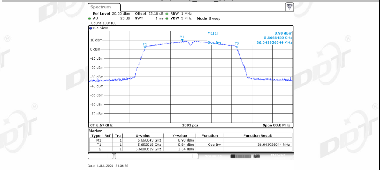
11AC40MIMO_Ant-3_5670
