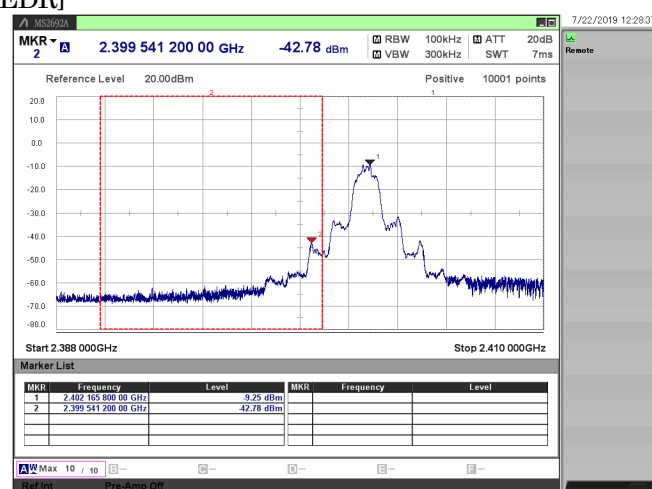
[EDR]
