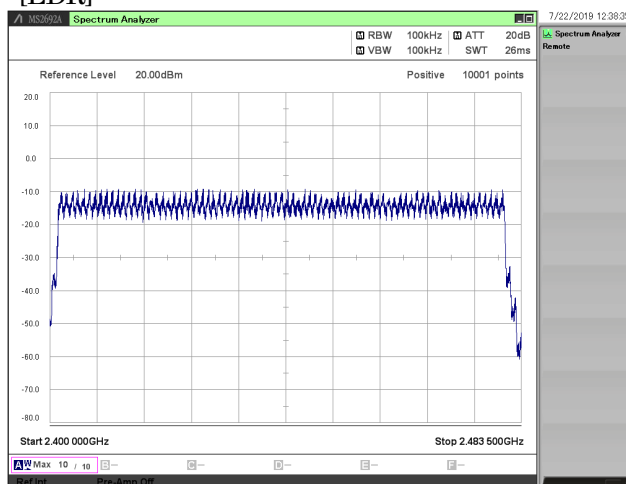
[EDR]
