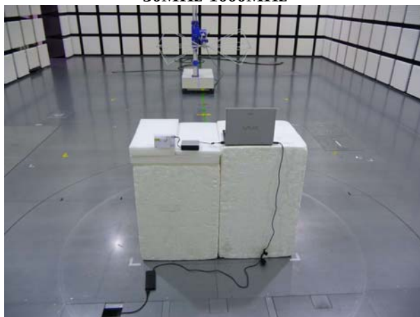
30MHz-1000MHz
