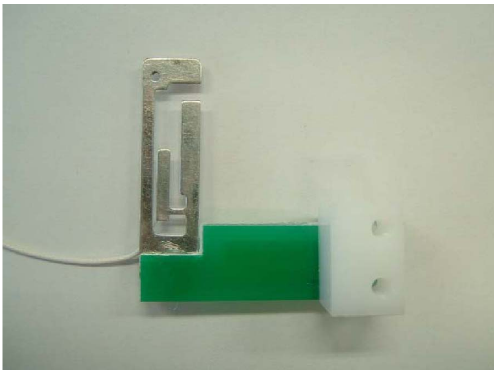
CAN4313359-REAR(Antenna)
