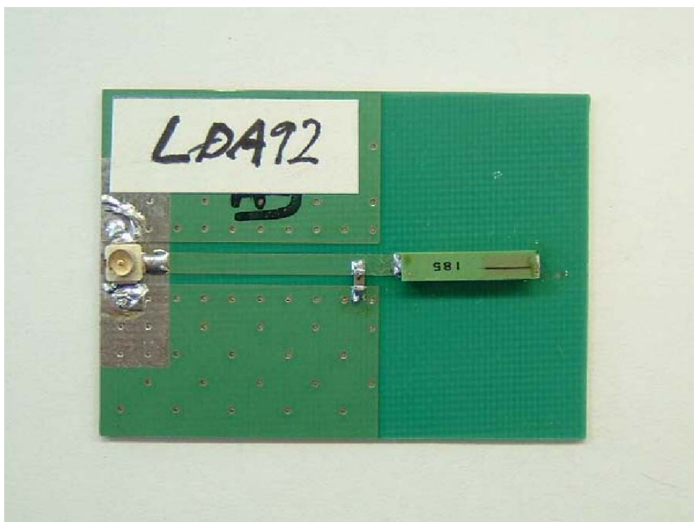
LDA92-FRONT(Antenna)
