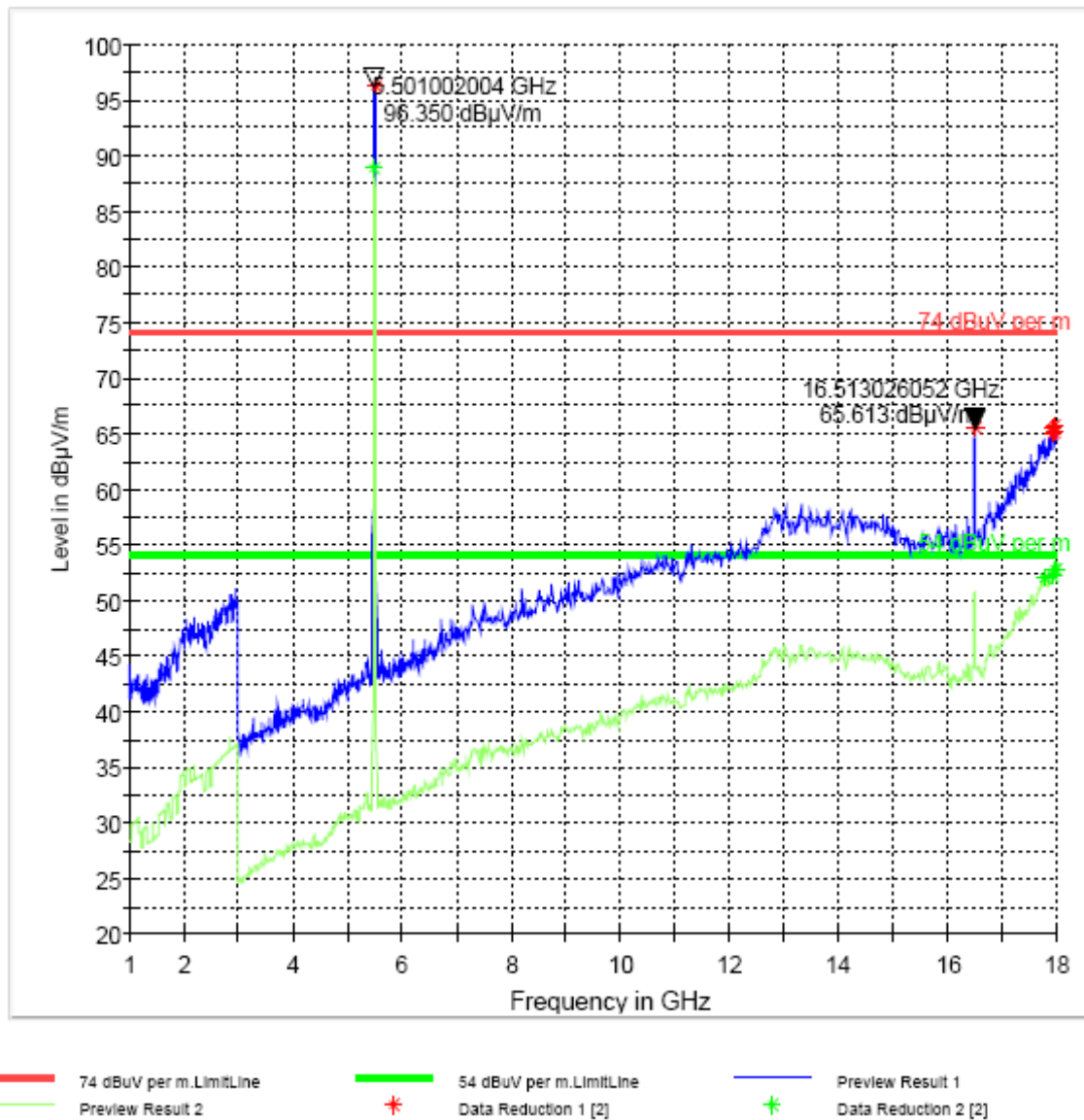
FCC 15 1-18GHz
