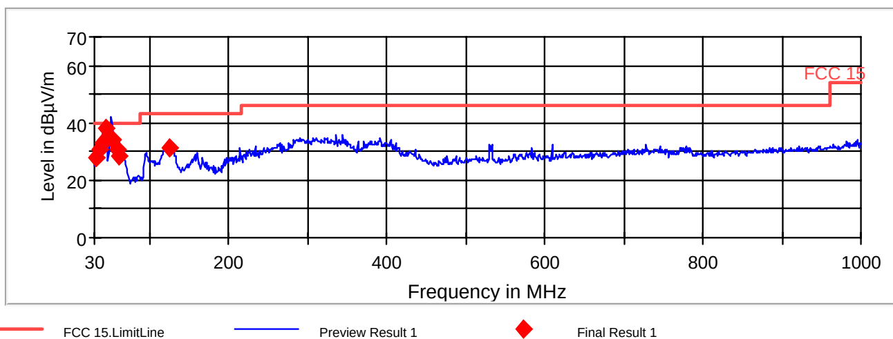
FCC 15 30-1000MHz
