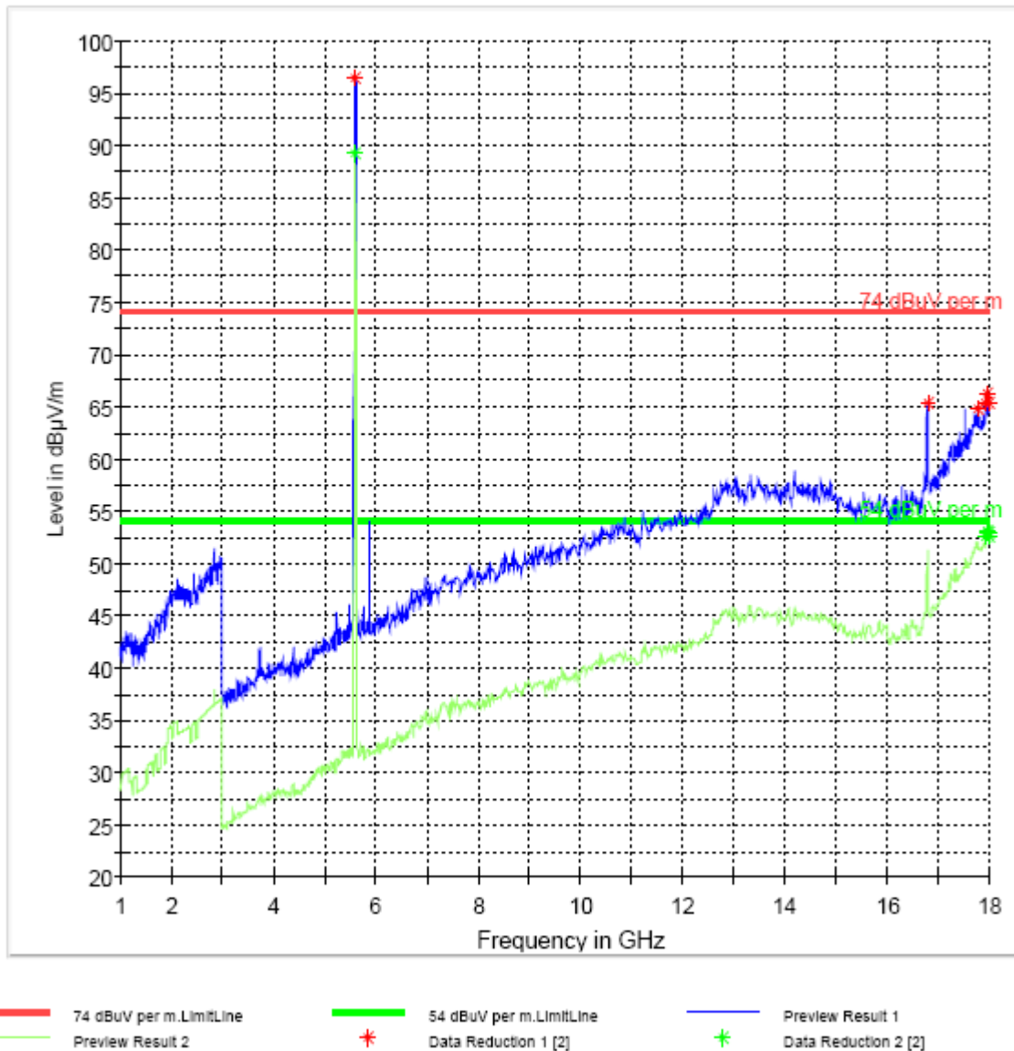
FCC 15 1-18GHz
