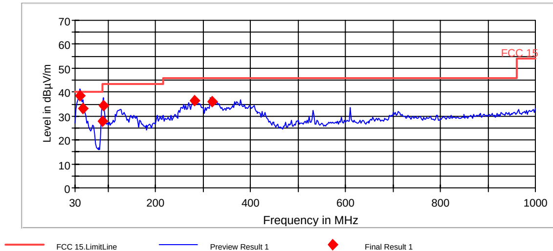
FCC 15 30-1000MHz
