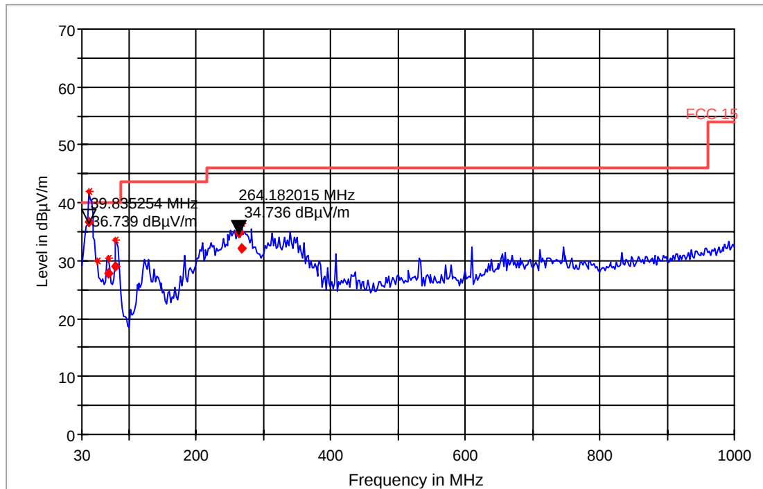
FCC 15 30-1000MHz
