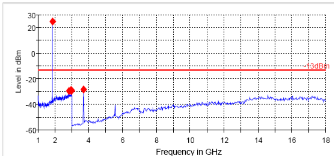
FCC 24 1-18GHz
