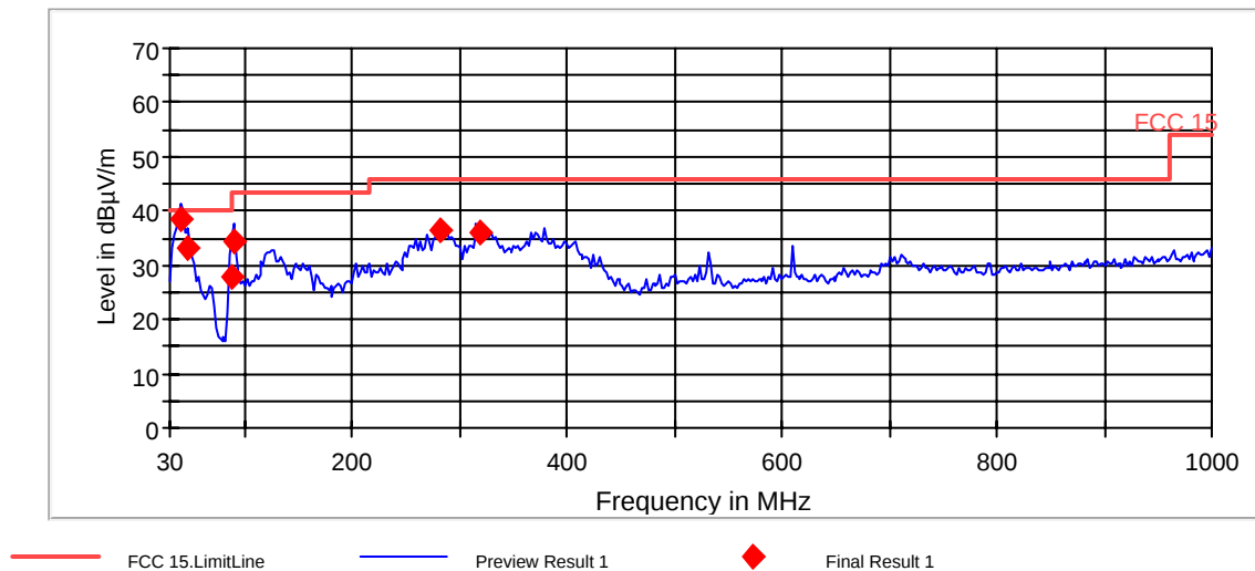
FCC 15 30-1000MHz
