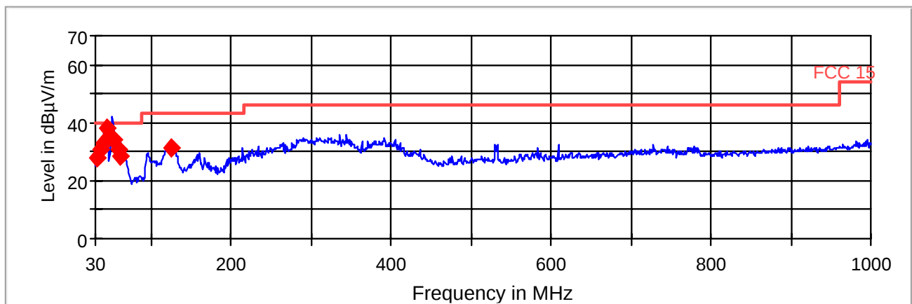
FCC 15 30-1000MHz
