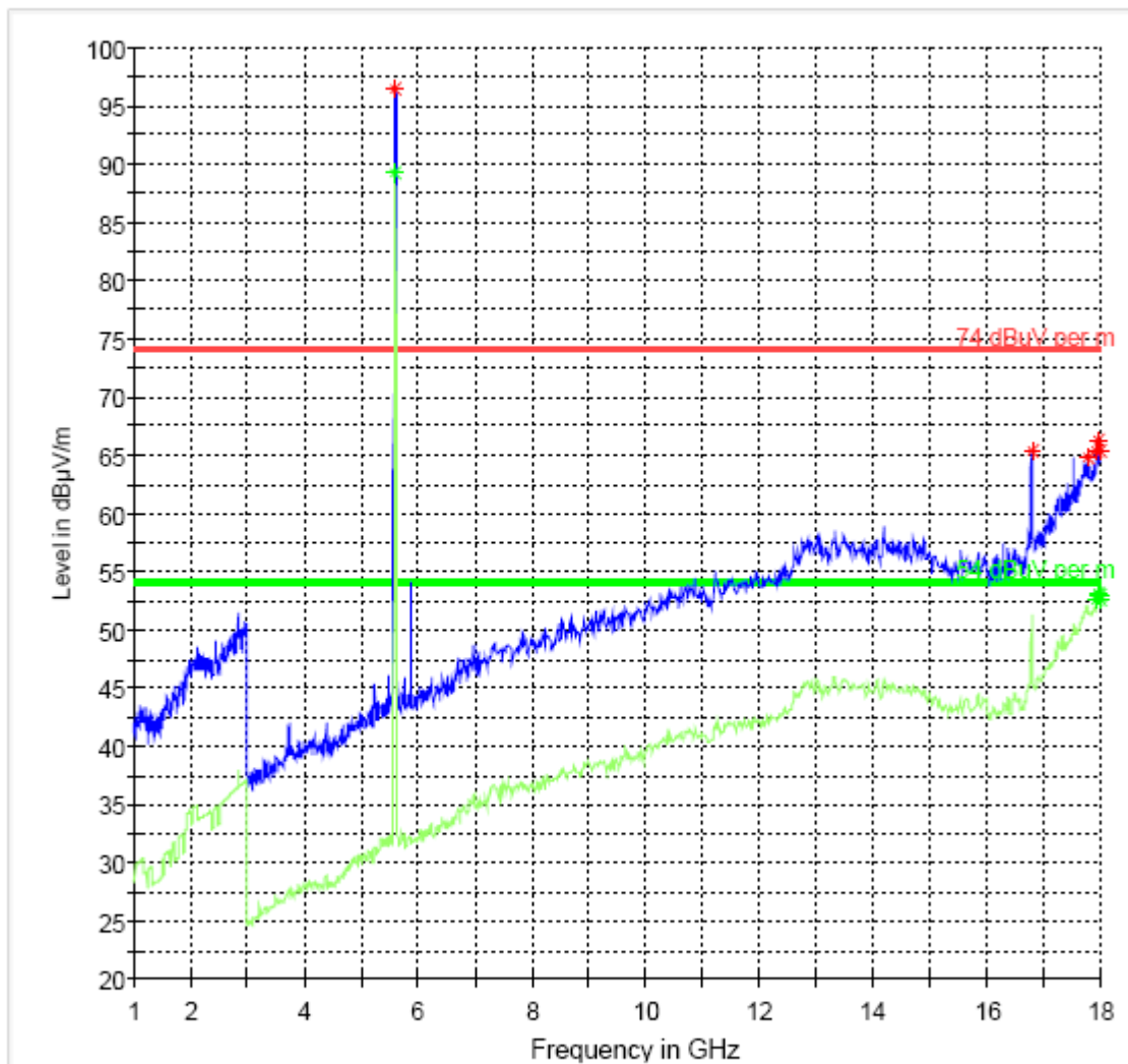
FCC 15 1-18GHz
