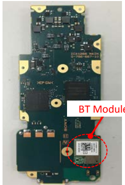
PWB IC side
