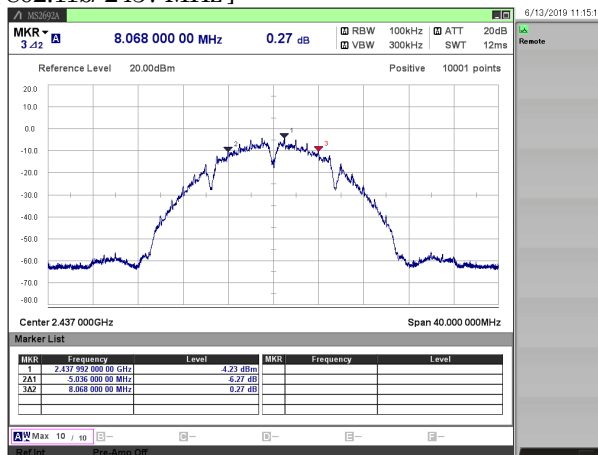
[ 802.11b/ 2437 MHz ]
