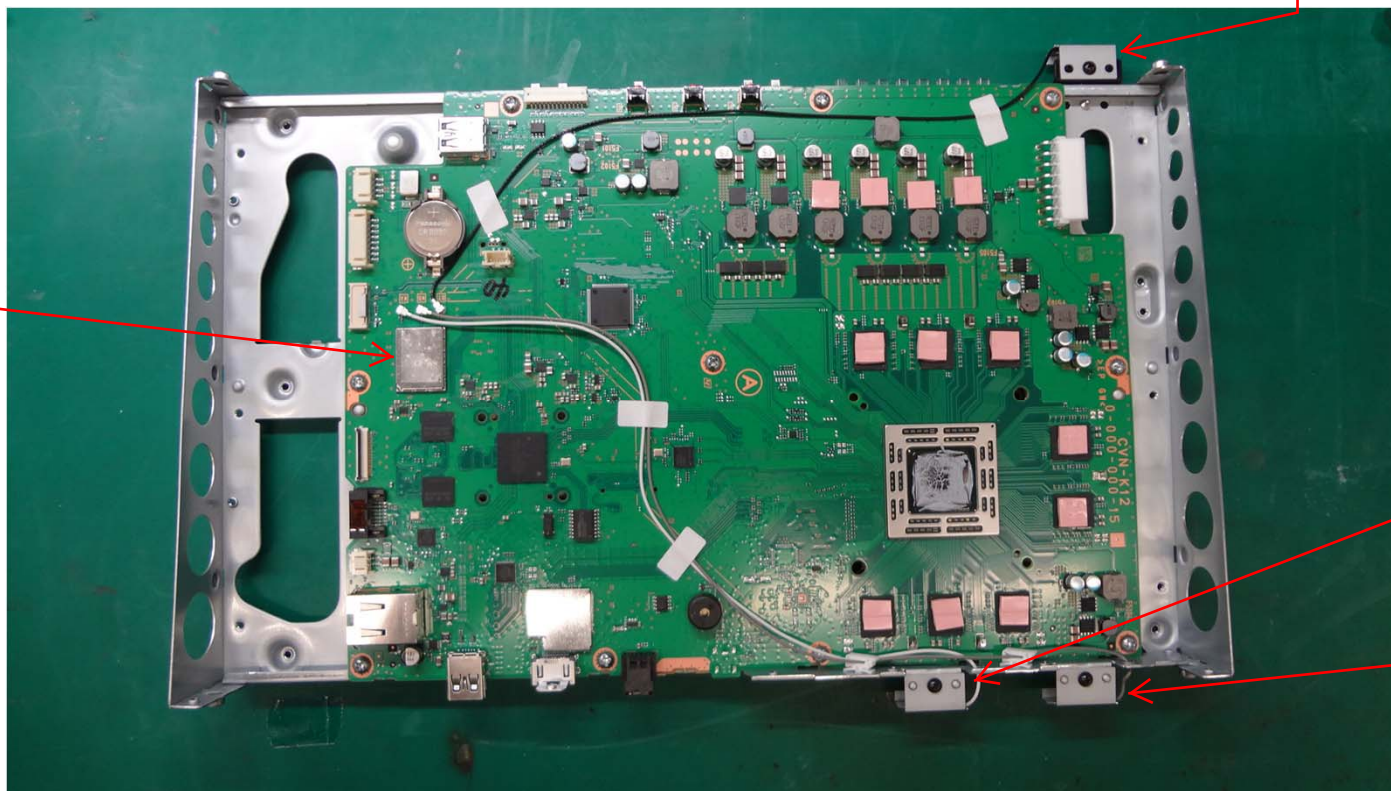
BT/WLAN module
