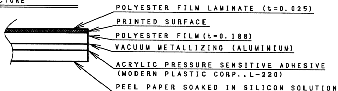
材料構成図 / COMPONENT MATERIAL STRUCTURE
