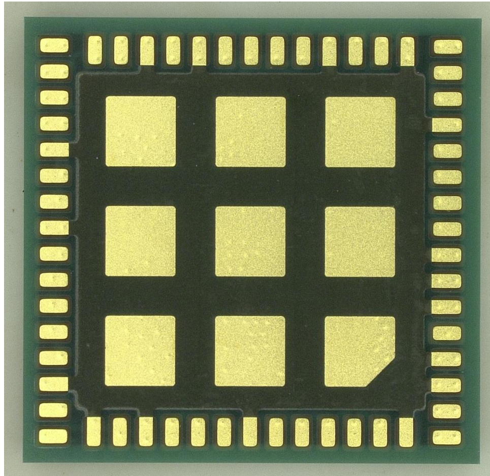
Module(Back)
