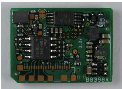
AES/DES UNIT(UT-134) SIDE A
