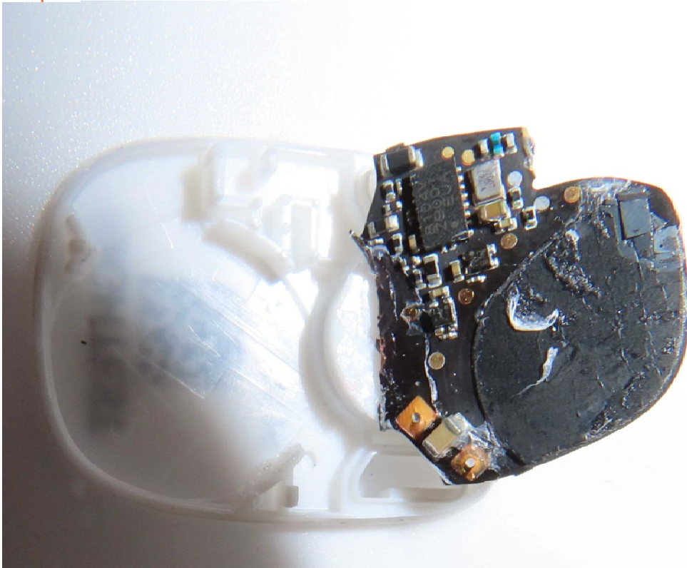
NFC Antenna
