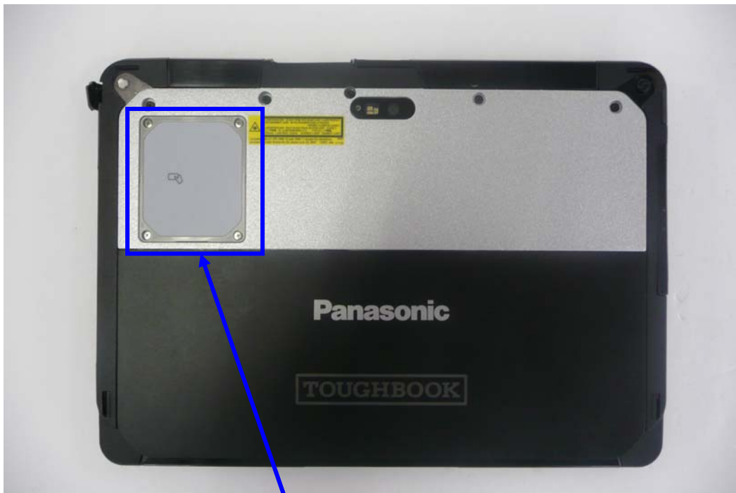
HF-RFID Module
