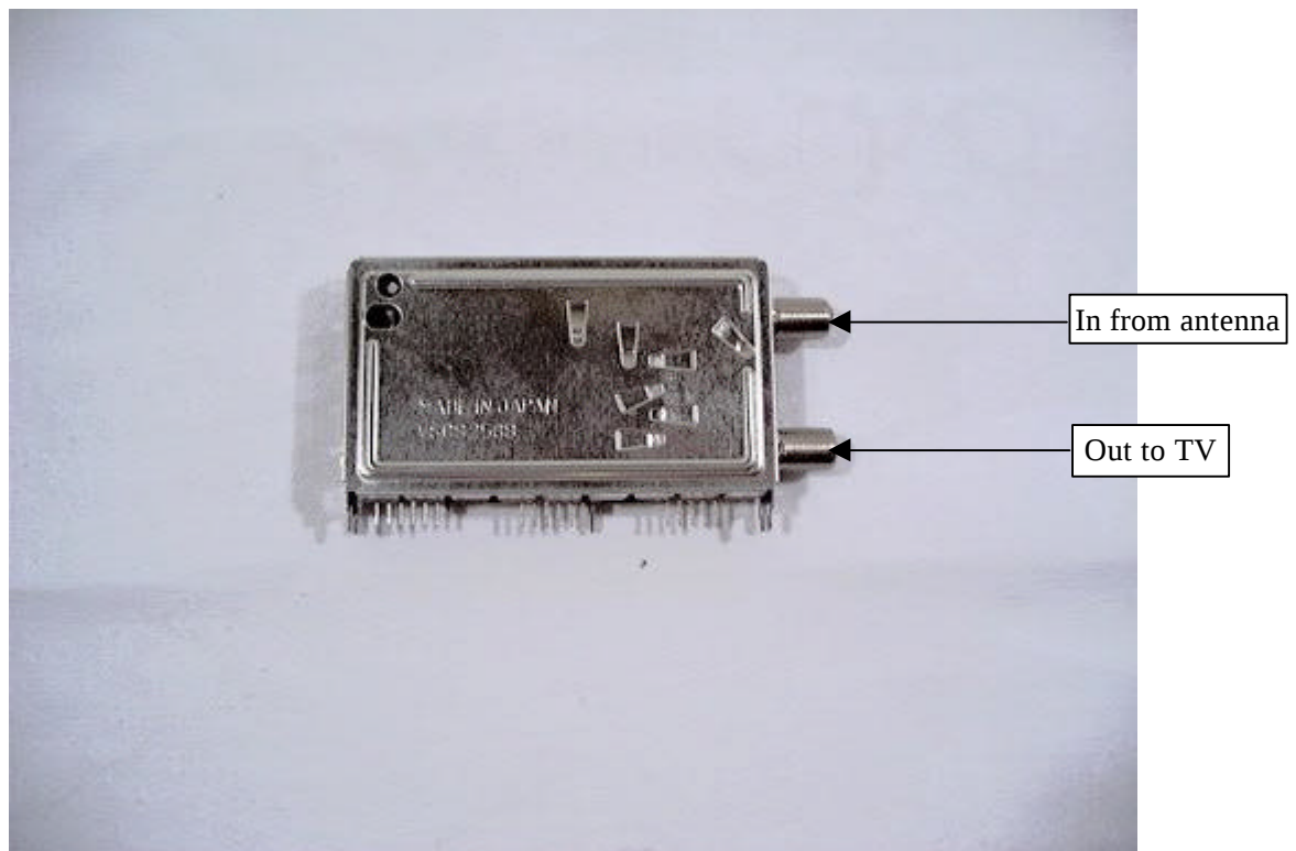
Tuner (VEQS0614: Top view)
