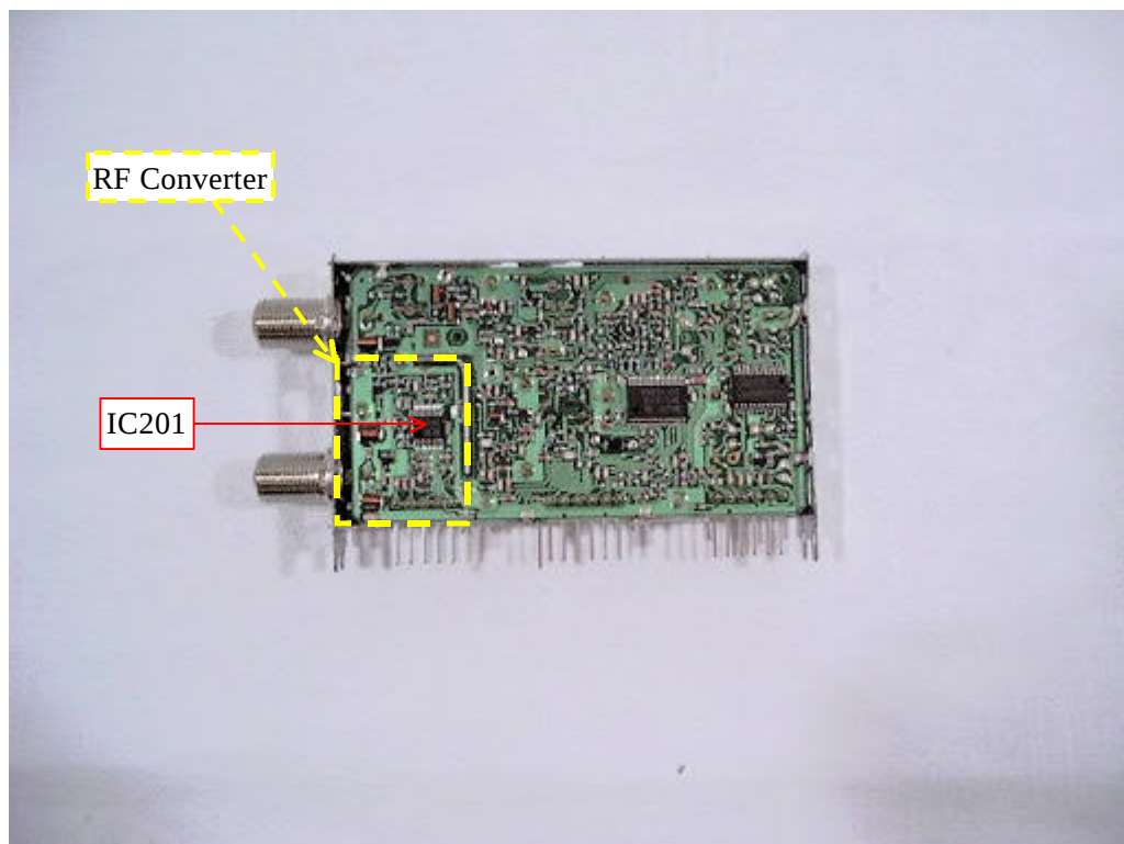
Tuner (VEQS0614: Bottom View)
