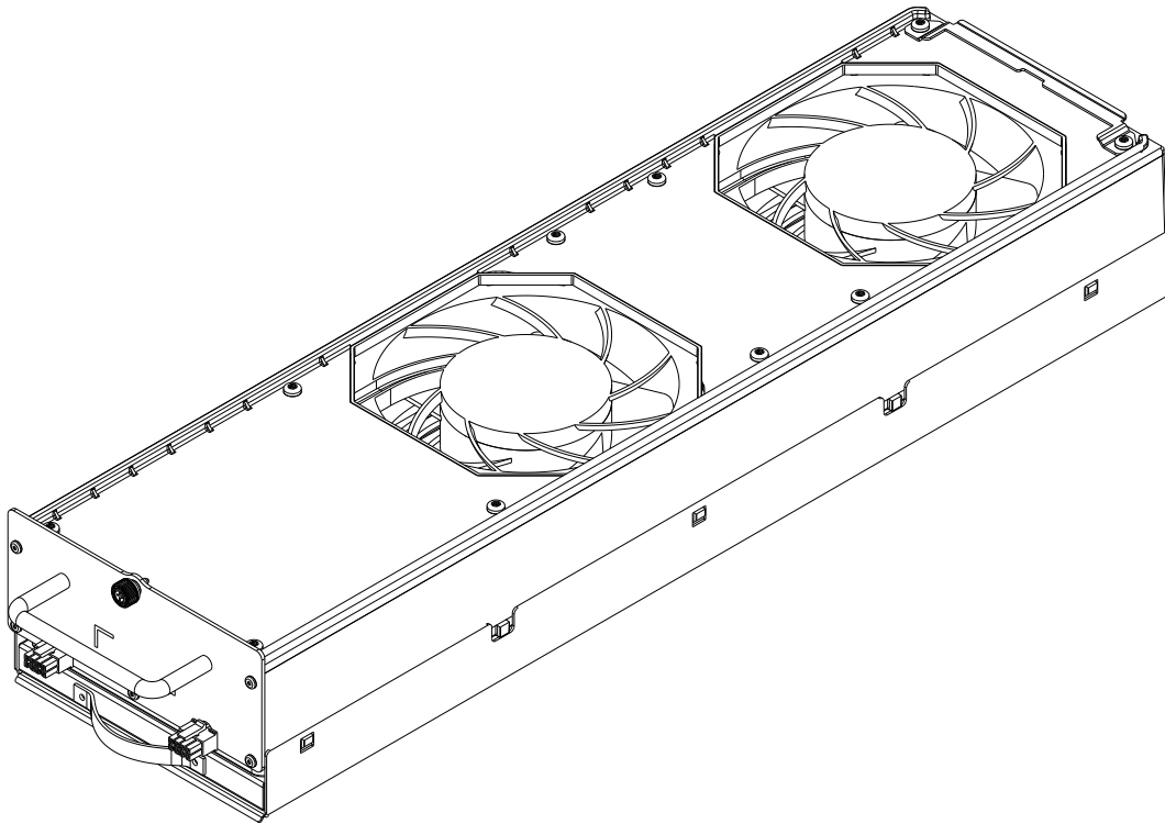
Figure 88: DSC 8500 Fan Assembly
