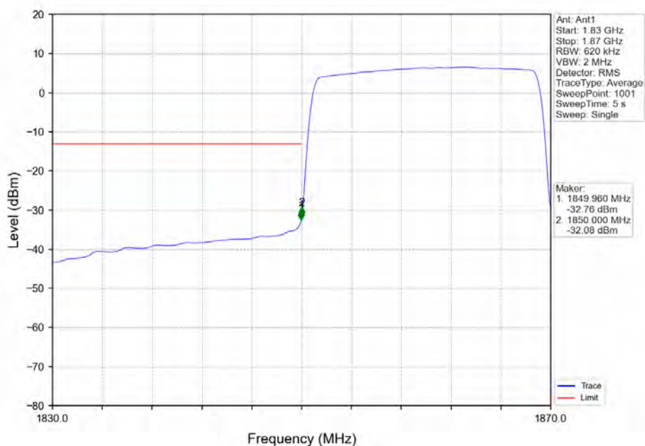
Band2_20MHz_16QAM_LCH_1860MHz_RB_100_0_NTNV
