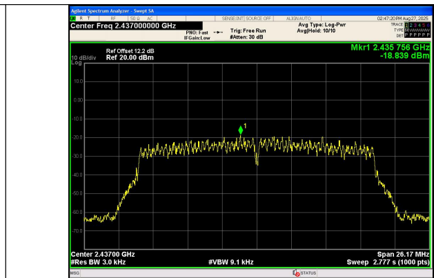
IEEE 802.11n_Channel 6_20MHz_Antenna 0
