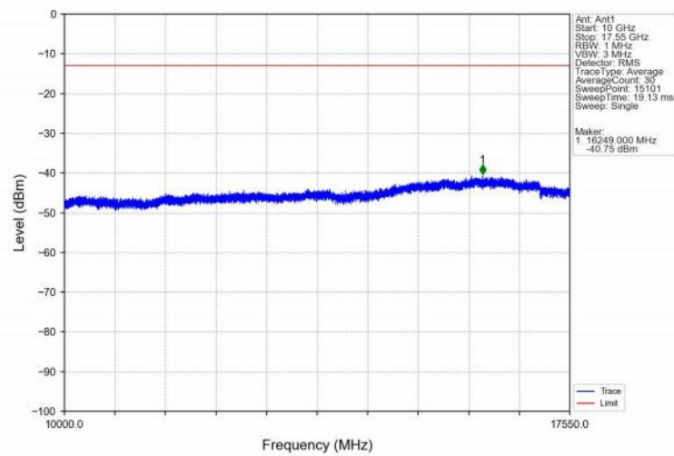
Band4_20MHz_QPSK_LCH_1720MHz_RB_1_0_NTNV
