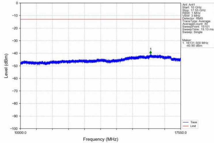
Band4_15MHz_QPSK_HCH_1747.5MHz_RB_1_74_NTNV
