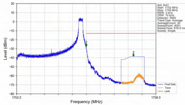
Band4_3MHz_QPSK_HCH_1753.5MHz_RB_1_14_NTNV
