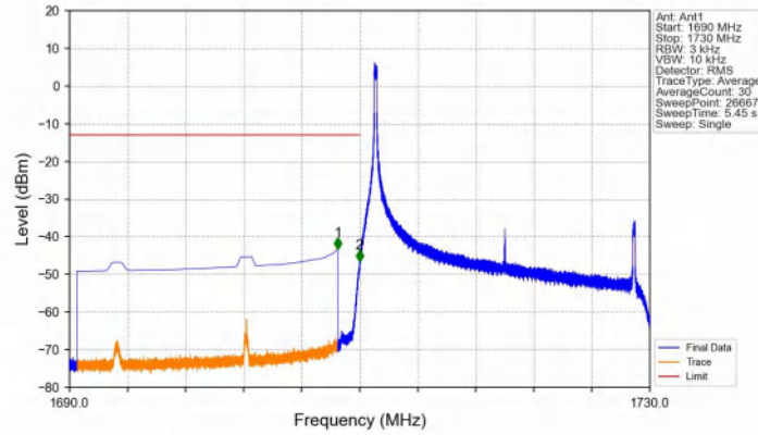
Band4_20MHz_QPSK_LCH_1720MHz_RB_1_0_NTNV
