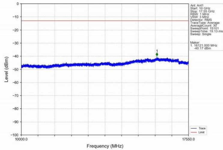
Band4_3MHz_QPSK_HCH_1753.5MHz_RB_1_14_NTNV
