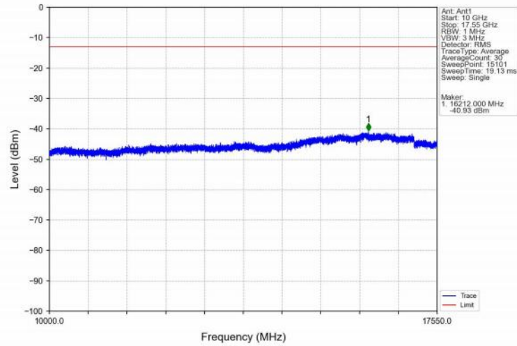
Band4_20MHz_QPSK_HCH_1745MHz_RB_1_99_NTNV
