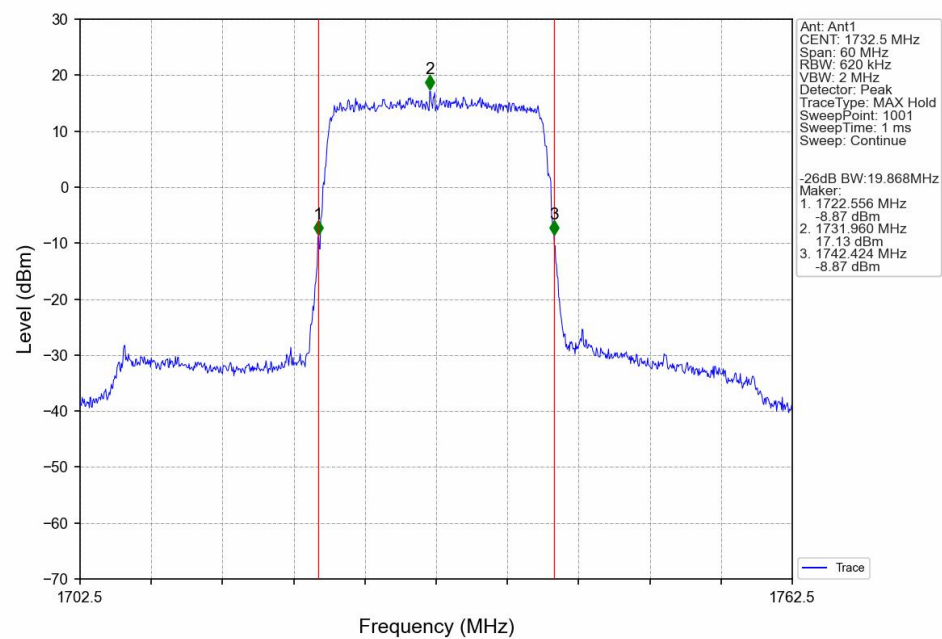
Band4_20MHz_QPSK_MCH_1732.5MHz_RB_100_0_NTNV
