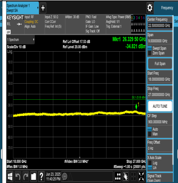
Band41-5MHz-QPSK-41565-1RB#0-18000~27000-PASS
