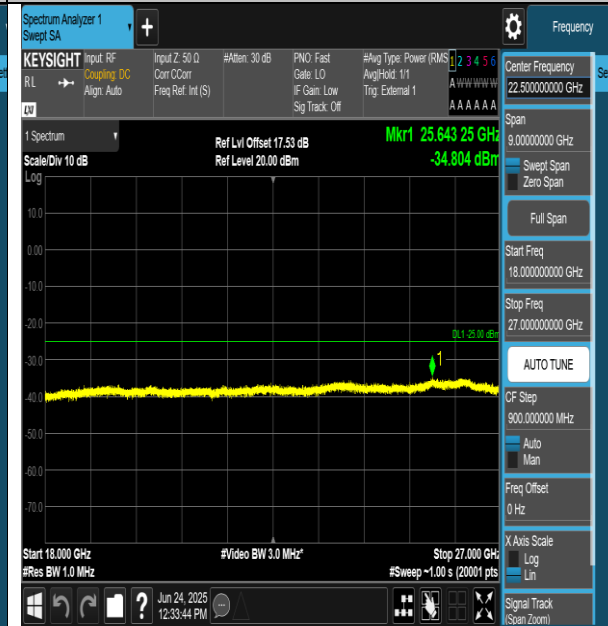
Band41-15MHz-QPSK-39725-1RB#0-18000~27000-PASS
