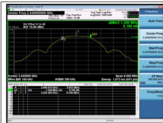
BLE 2Mbps 2440MHz -6dB BW
