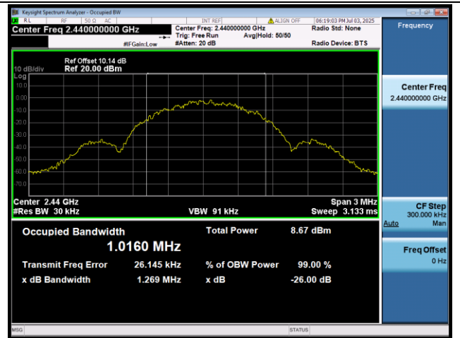
BLE 1Mbps 2440MHz 99% OBW
