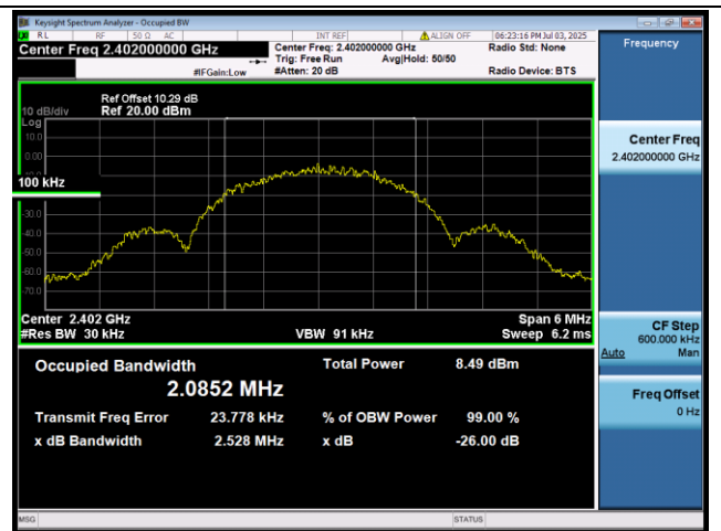
BLE 2Mbps 2402MHz 99% OBW
