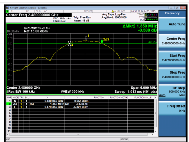
BLE 2Mbps 2480MHz -6dB BW
