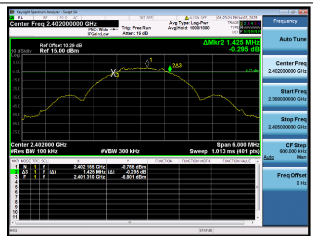
BLE 2Mbps 2402MHz -6dB BW
