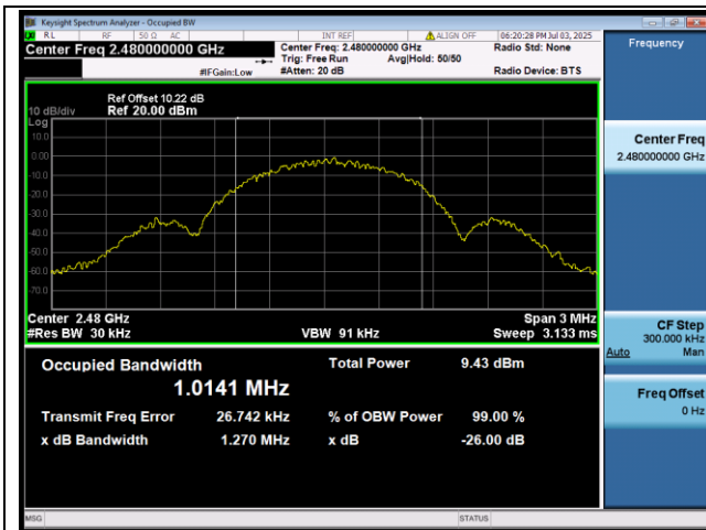
BLE 1Mbps 2480MHz 99% OBW
