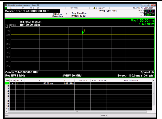
BLE 1Mbps 2440MHz
