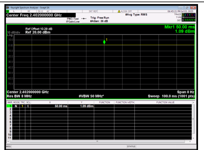
BLE 2Mbps 2402MHz
