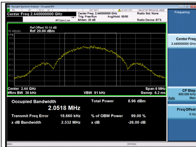
BLE 2Mbps 2440MHz 99% OBW
