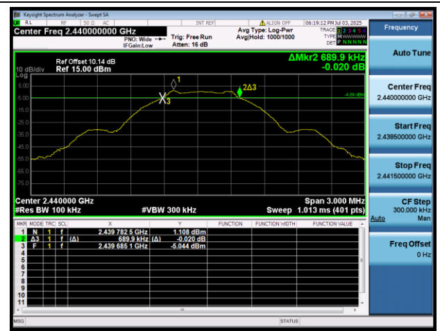
BLE 1Mbps 2440MHz -6dB BW
