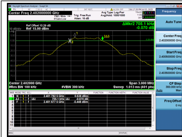
BLE 1Mbps 2402MHz -6dB BW
