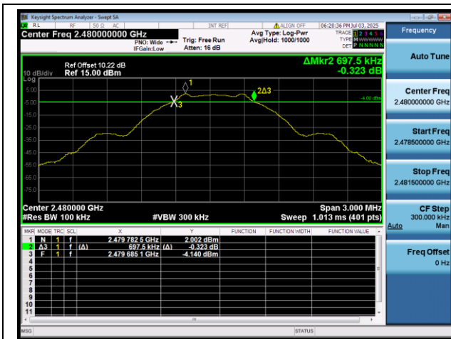
BLE 1Mbps 2480MHz -6dB BW
