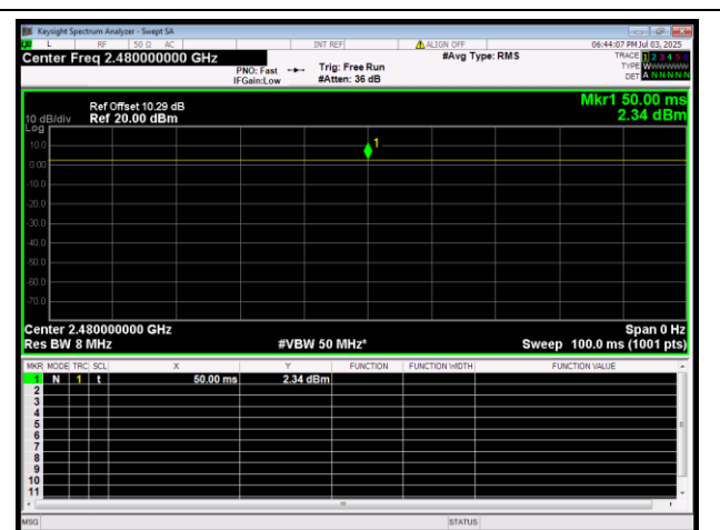
BLE 2Mbps 2480MHz
